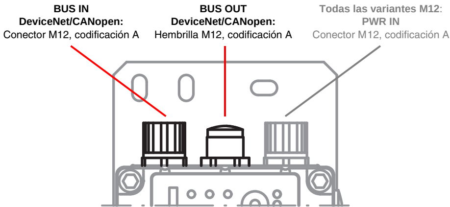
Figura 9.6: Posición y denominación de las conexiones M12 DeviceNet/CANopen
