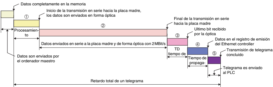
Figura 10.11: Típica estructura de telegrama Ethernet
