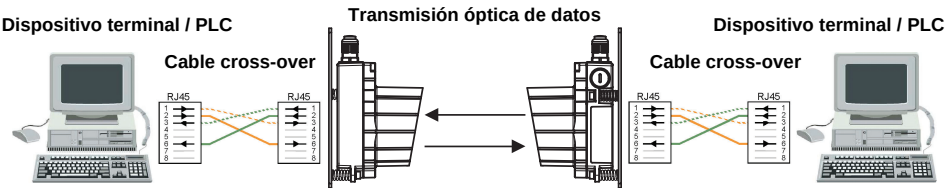
Figura 10.7: DDLS 200 entre dispositivo terminal/PLC y dispositivo terminal/PLC
