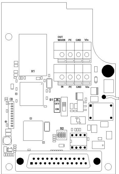
Figura 10.1: Placa de conexión modelo Ethernet
