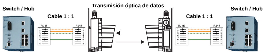
Figura 10.6: DDLS 200 entre switch/hub y switch/hub
