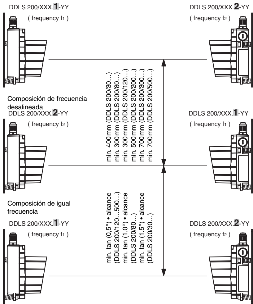
Figura 4.2:Disposición de sistemas de transmisión vecinos
