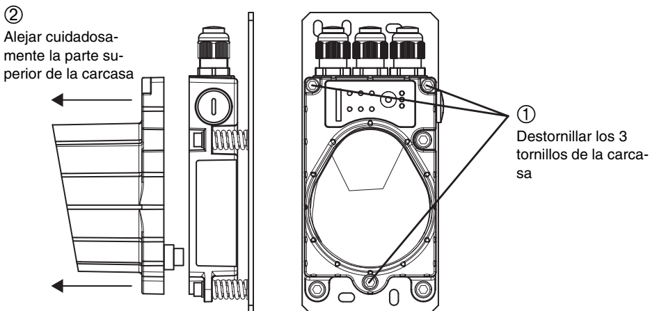
Figura 4.4: Quitar la parte superior de la carcasa
