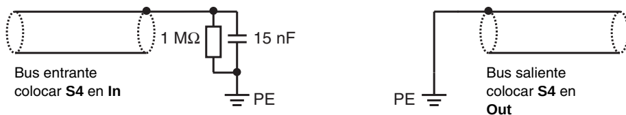
Figura 6.3: Conexión de blindaje en bus entrante/ saliente
