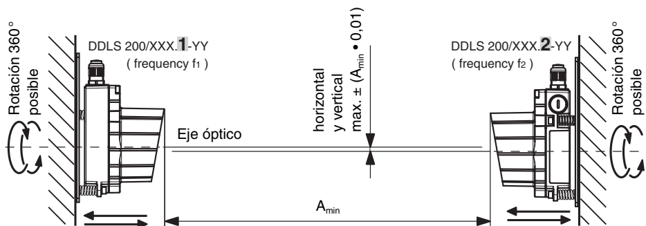
Figura 4.1: Montaje de los equipos
