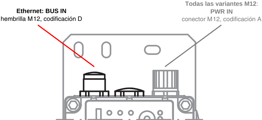
Figura 10.2: Posición y denominación de los conectores M12 Ethernet
