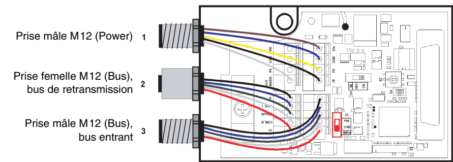
Figure 9.5: Montage et raccordement des connecteurs M12 en option
