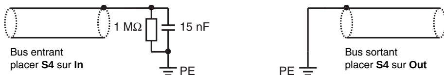
Figure 6.3: Blindage pour le bus entrant/sortant
