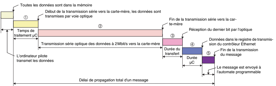
Figure 10.11 :Structure typique du message Ethernet
