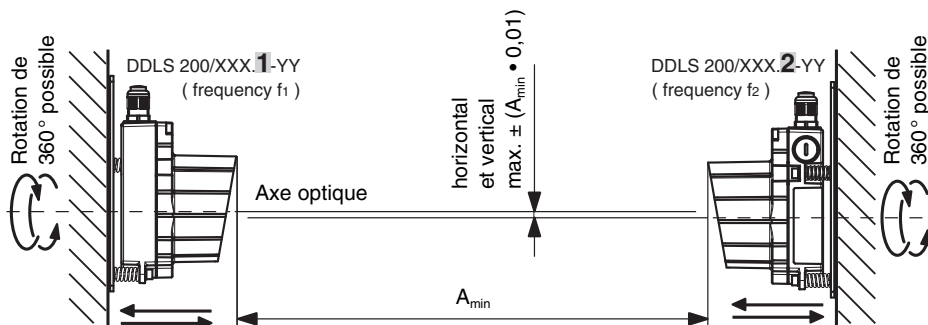
Figure 4.1: Montage des appareils
