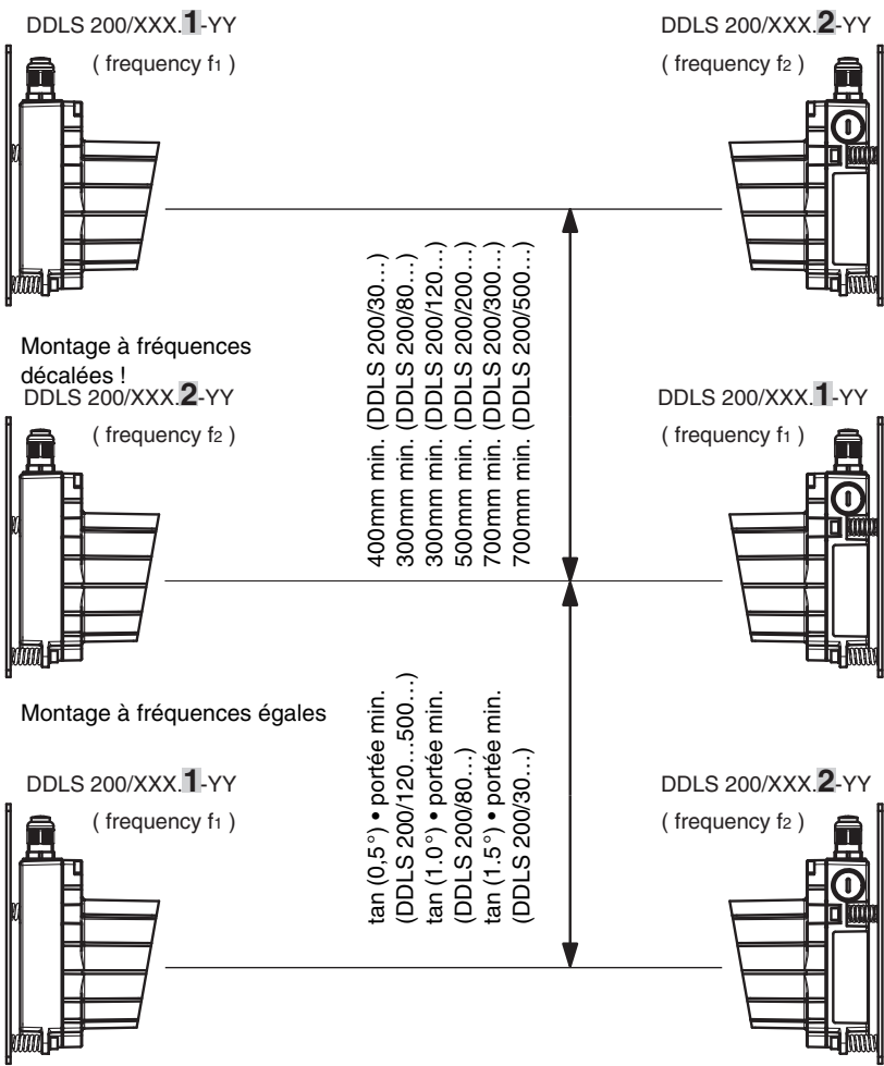
Figure 4.2: Disposition de systèmes de transmission voisins
