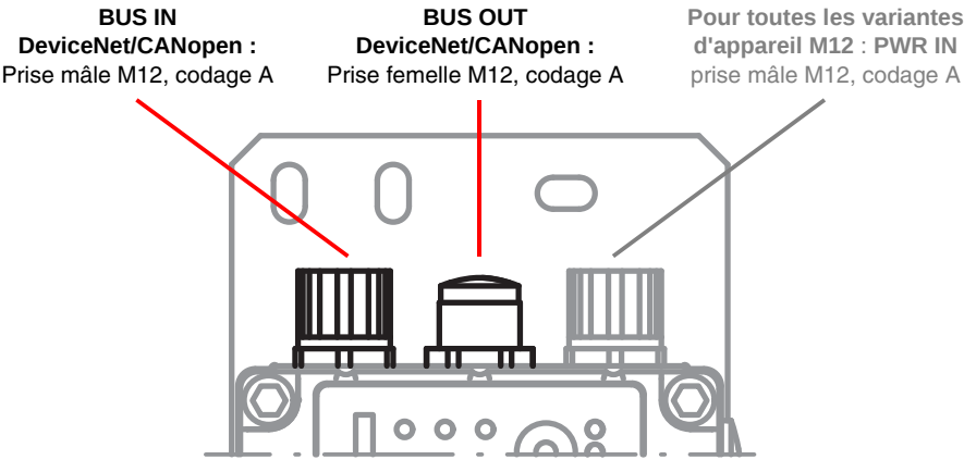
Figure 9.6: Emplacement et désignation des ports DeviceNet/CANopen M12
