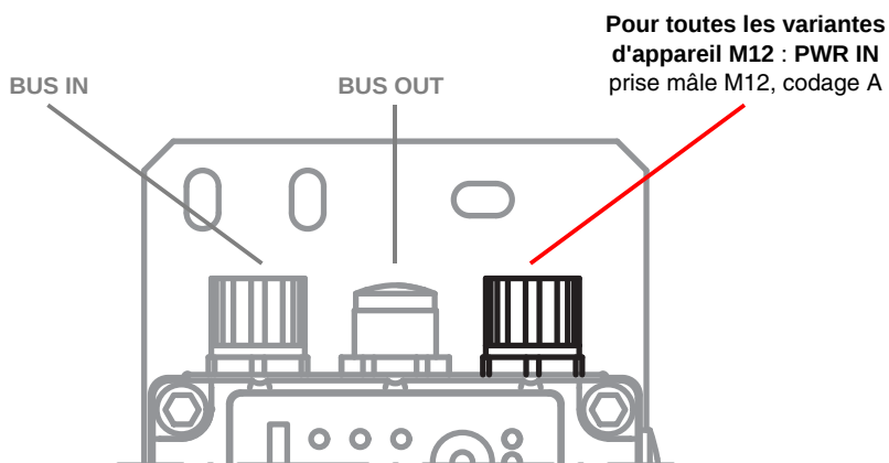
Figure 4.6: Emplacement et désignation des ports M12
