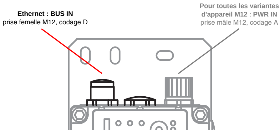
Figure 10.2 : Emplacement et désignation des ports Ethernet M12
