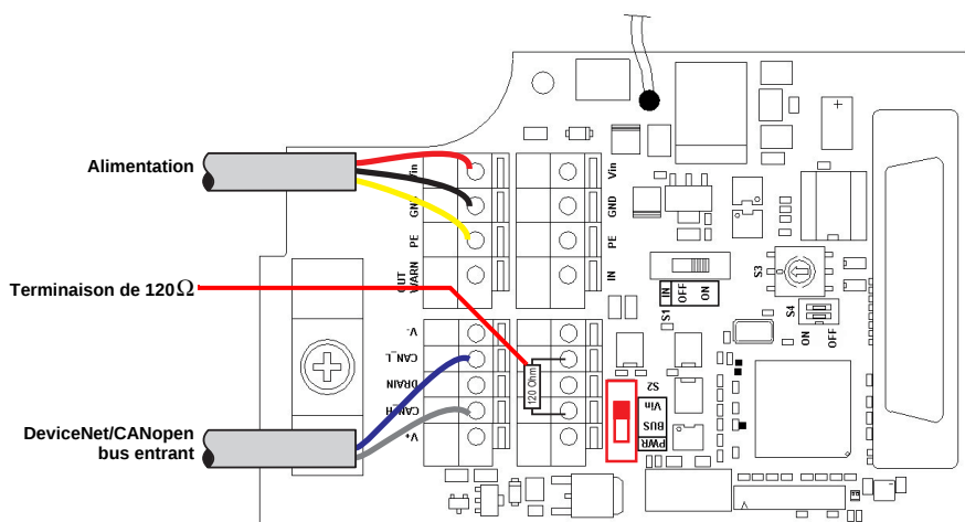
Figure 9.10: Terminaison dans l'appareil
