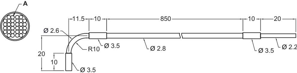
A Ø 0.265 mm プラスチック繊維芯 x 32 個
