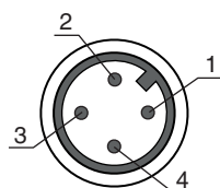
Figura 5.1: Occupazione dei pin del trasmettitore
