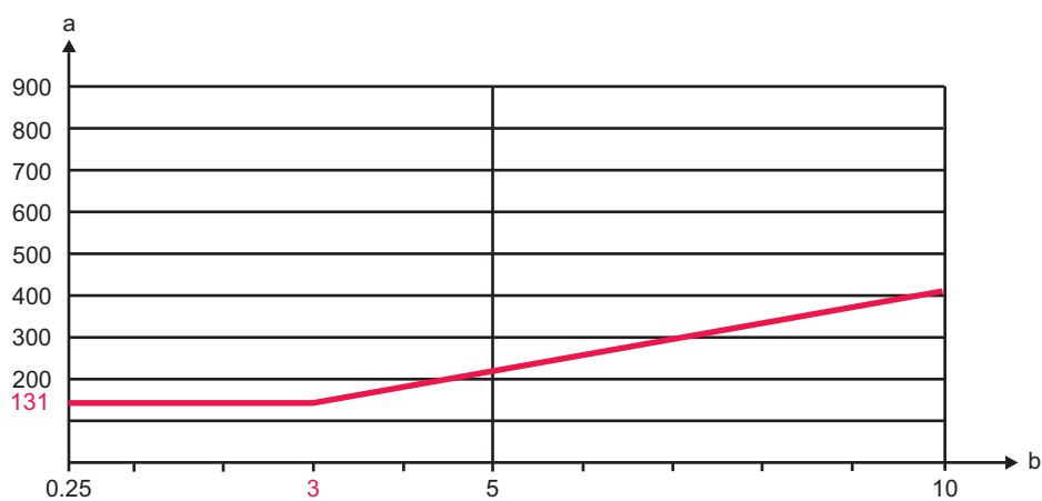
Figura 4.2: Distanza minima fino alle superfici riflettenti
