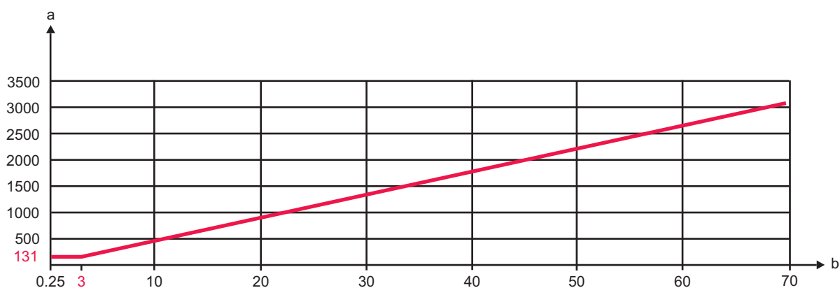
Figura 4.3: Distanza minima fino alle superfici riflettenti in funzione della larghezza del campo protetto fino a 10 m
