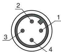
Figura 5.2: Occupazione dei pin del ricevitore
