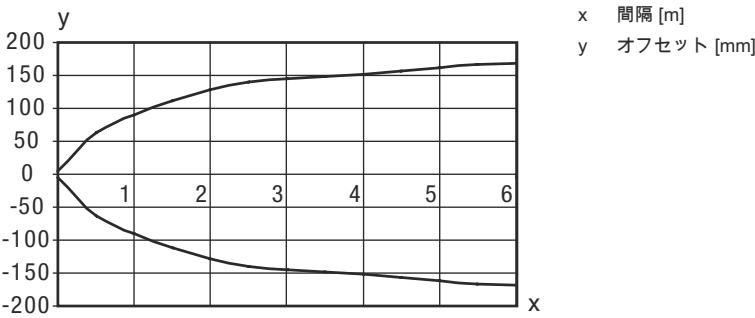
典型的な応答動作 ( TKS100x100 )
