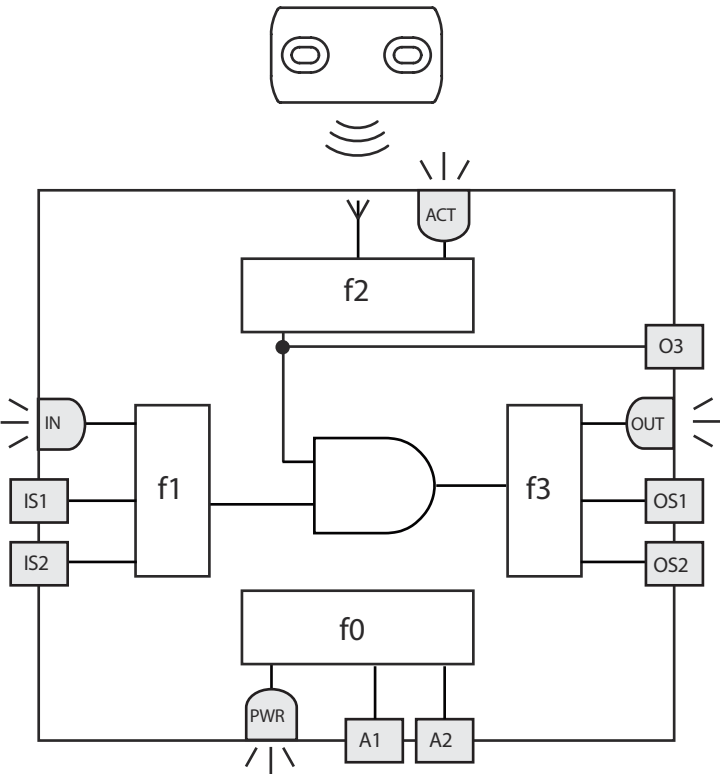
Schéma des connexions internes
