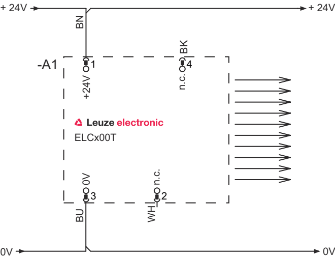
송신기 연결도
