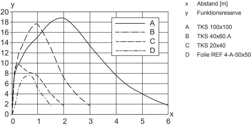
Typ. Funktionsreserve
