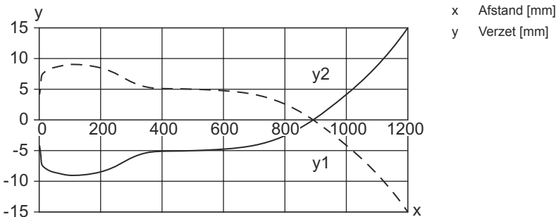
Typisch aanspreekgedrag (instelafstand 1200 mm)
