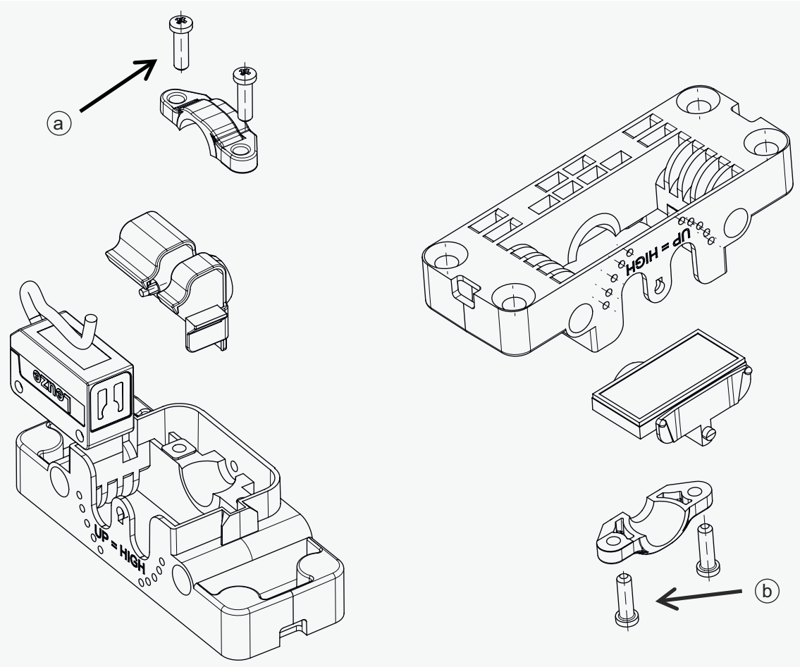
a 松开螺栓以校准传感器 b 松开螺栓以校准反射器
