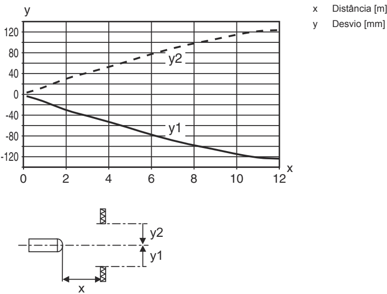
Comportamento de resposta típ. (TKS100x100)
