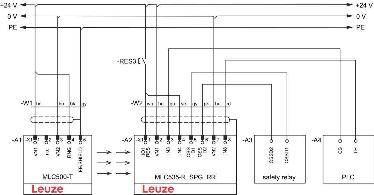
运行模式 5：含智能过程门控 (SPG) 的接线示例
