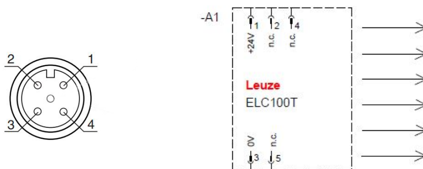
Figura 6.1: Assegnazione dei pin e schema di collegamento trasmettitore
