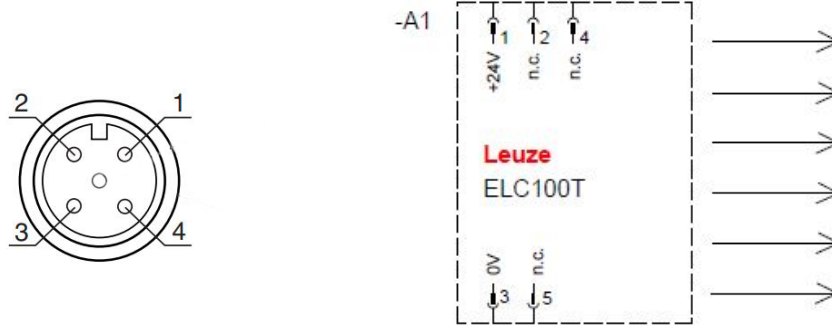
Resim 6.1: Vericinin pim tahsisi ve bağlantı şeması
