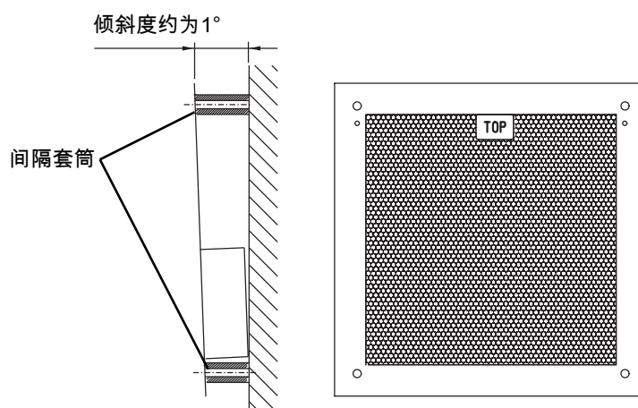
图 5.13: 加热反射器的倾斜
