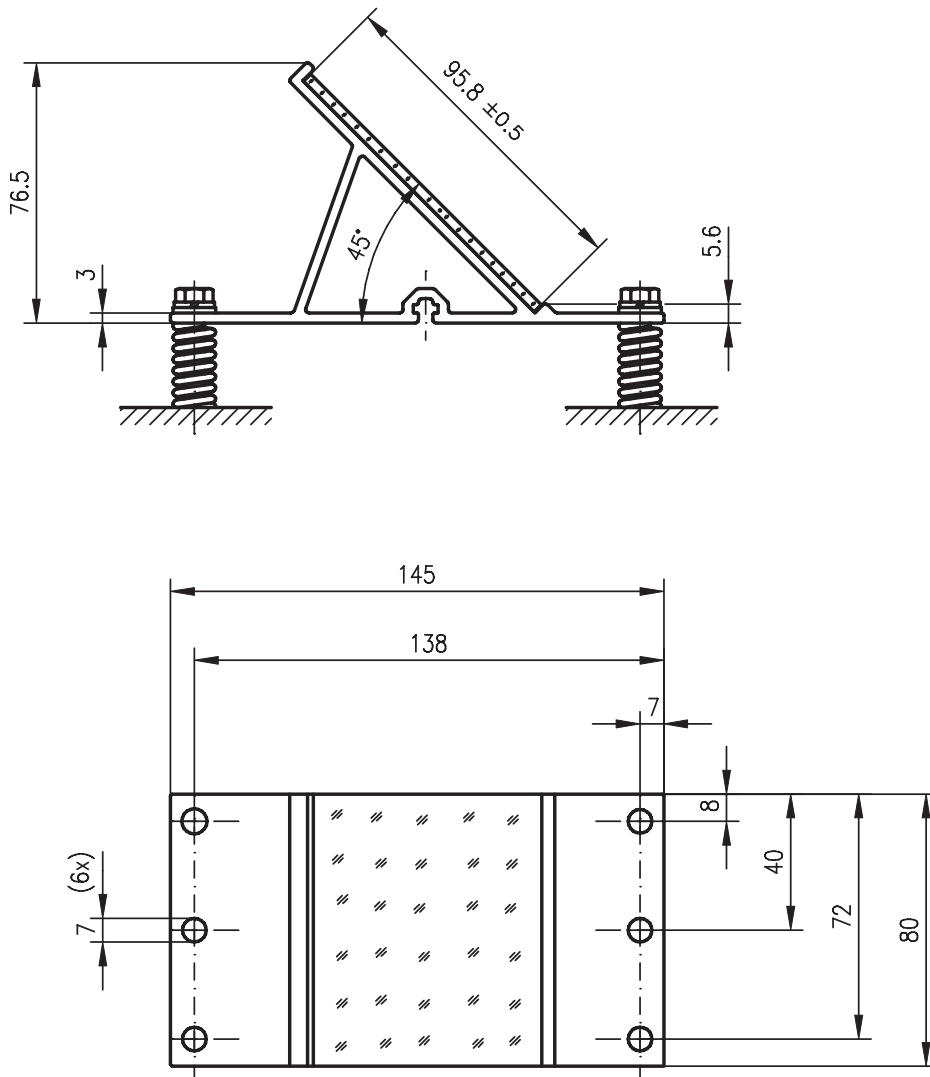
偏转单元 US 1 OMS
