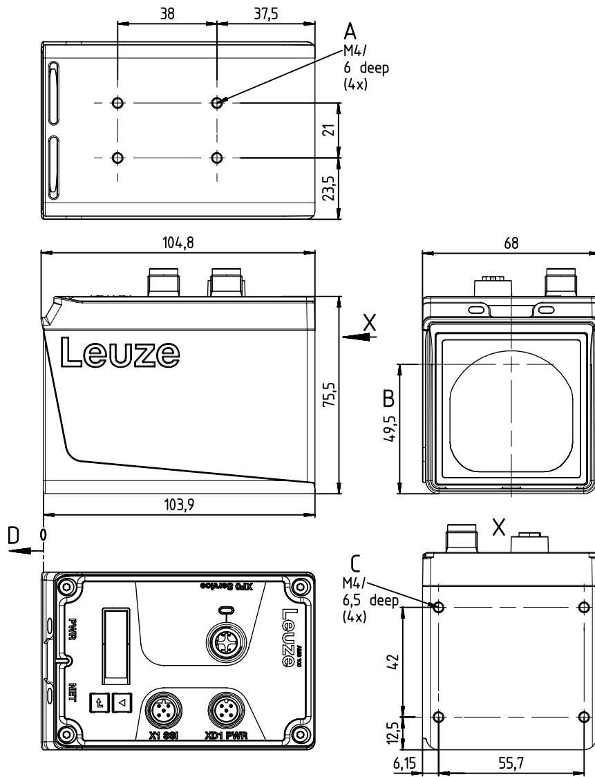
图 11.1: AMS 107i 光学激光测量系统
