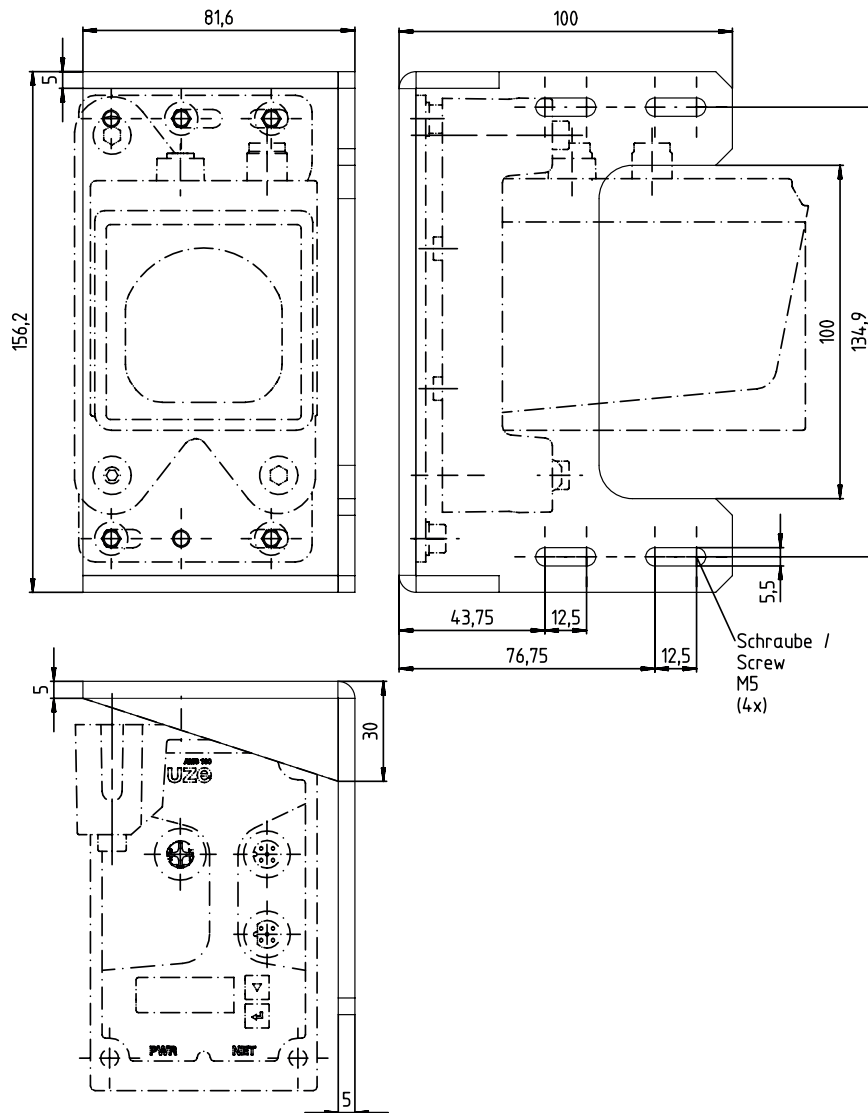
图 11.4: 安装设备 BT 0100M-F · 用于地面安装或水平面
