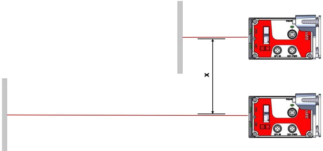
图 5.7: 移动反射器的平行安装
