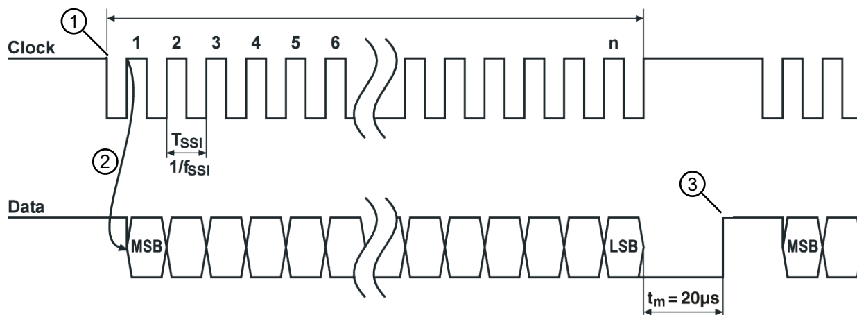
图 7.1: SSI 传输周期
