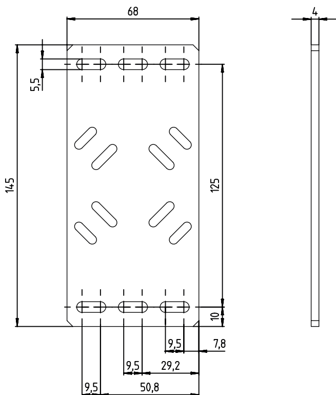
图 11.3: 安装设备 BT 0100M，用于在没有校准单元的情况下安装
