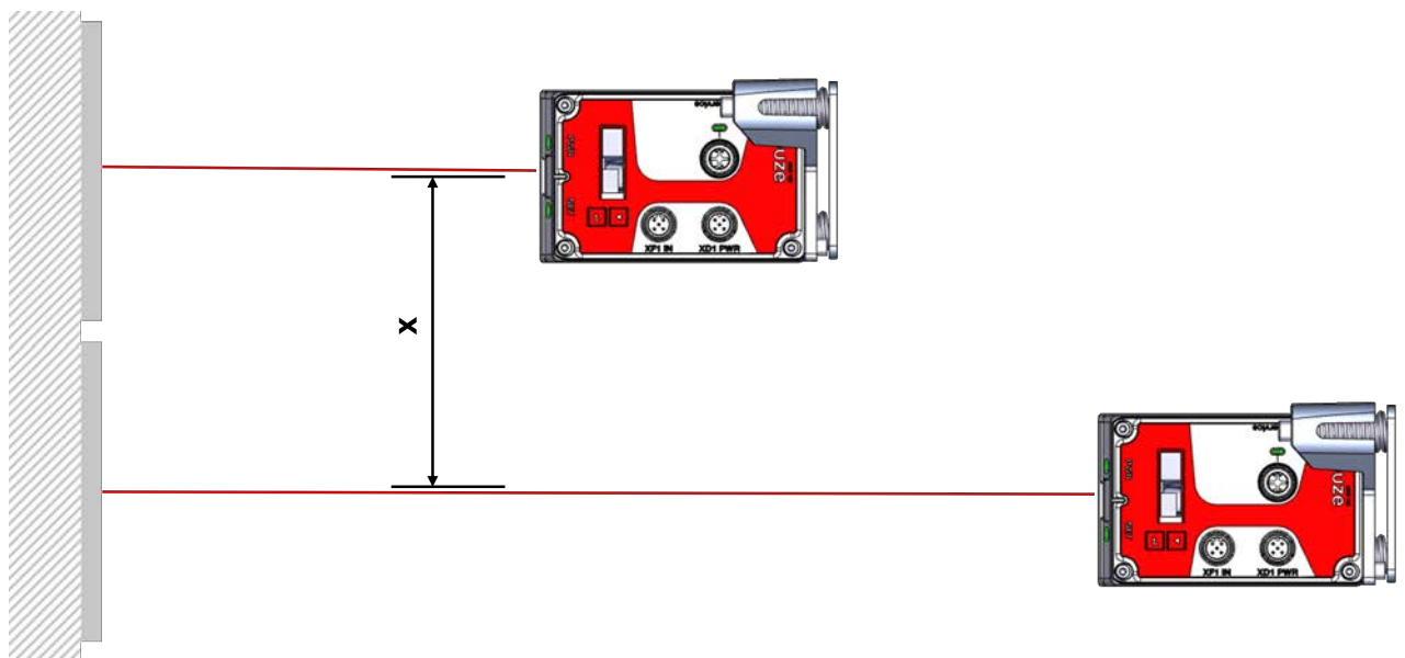
图 5.8: 移动 AMS 100i 的平行安装
