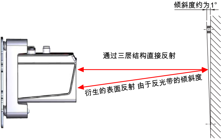
图 5.10: 反射器安装
