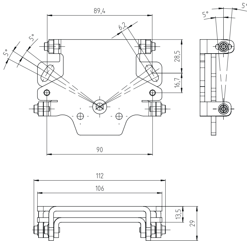
그림 14.4: 설치 시스템 BTU 500M
