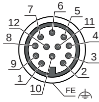
그림 7.2: M12 커넥터(12핀) 핀 지정
