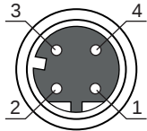
그림 7.3: 이더넷 인터페이스 핀 지정
