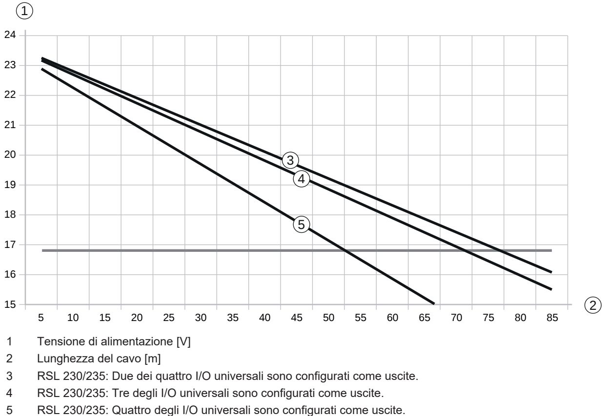
Figura 7.1: Schema per la stima della caduta di tensione sul cavo di alimentazione (sezione del cavo = 0,14 mm 2 (cavo a 12 pin))
