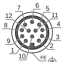
Figura 7.2: Assegnazione dei pin del connettore maschio M12, a 12 poli
