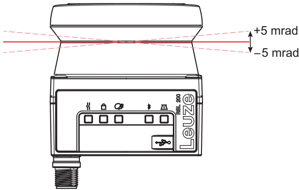
Figura 14.2: Error de inclinación
