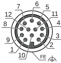
Bild 7.2: Pinbelegung M12-Stecker, 12-polig
