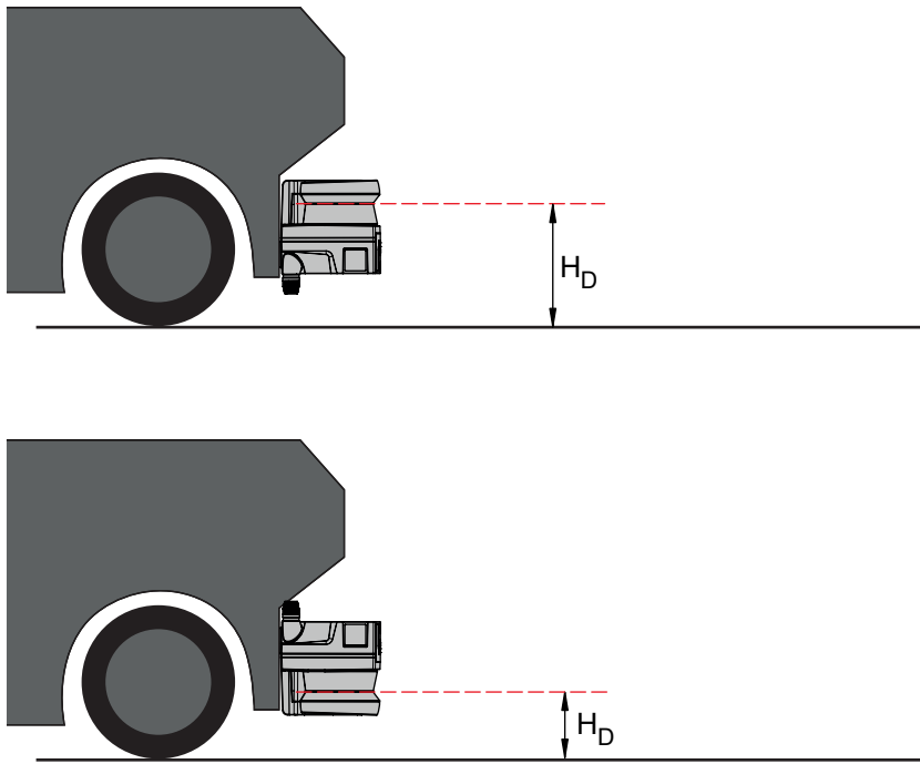
Bild 6.12: Empfohlene Montagehöhe H_D für RSL 210, RSL 220 und RSL 230 bei fahrerlosen Transportsystemen (Nutzung der Sicherheitsfunktion)
