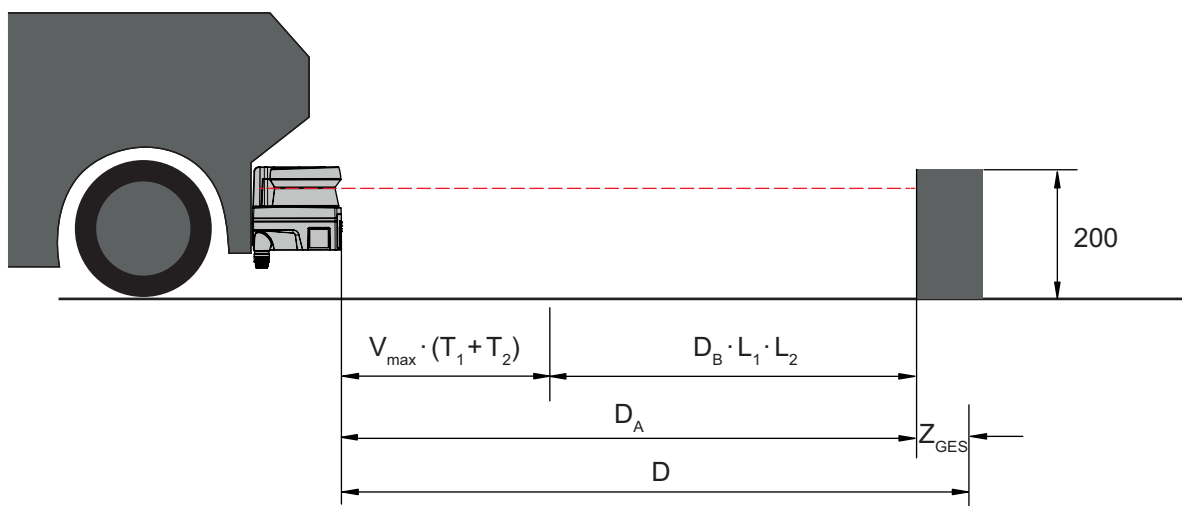
Bild 6.14: Mobile Gefahrbereichssicherung, Berechnung der erforderlichen Mindestdistanz D
