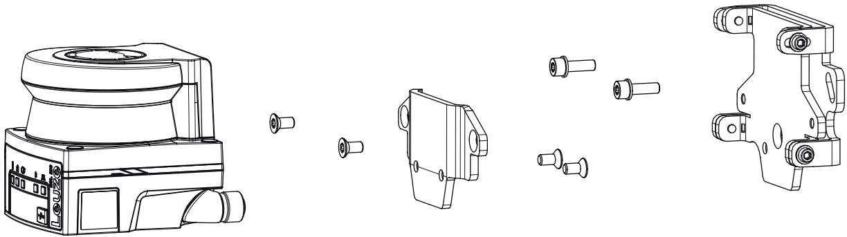
Bild 6.17: Montage mit Wandhalter
