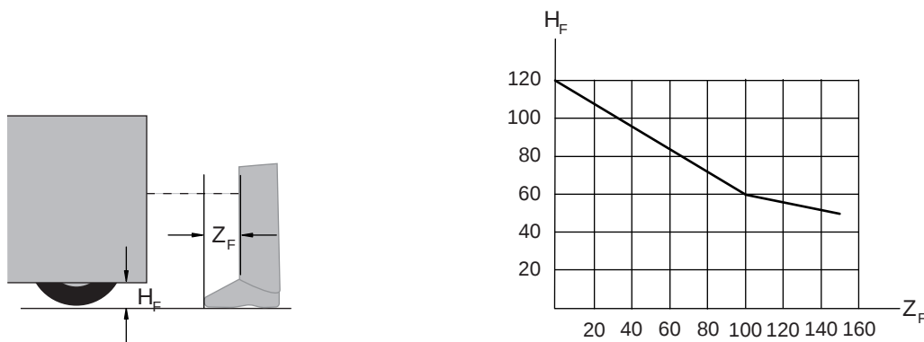
Bild 6.15: Diagramm zur Bestimmung des Zuschlags Z_{\text{F}} bei mangelnder Bodenfreiheit H_{\text{F}}
