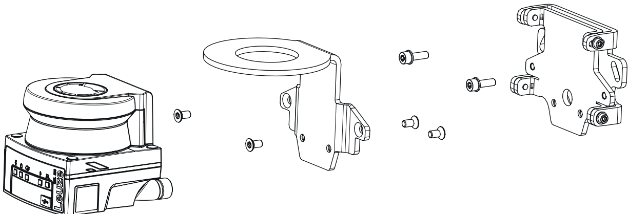
Bild 6.18: Montage mit Wandhalter und Schutzbügel
