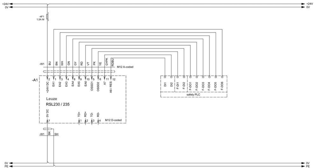
Bild 7.4: RSL 230/235 mit Sicherheits-Steuerung
