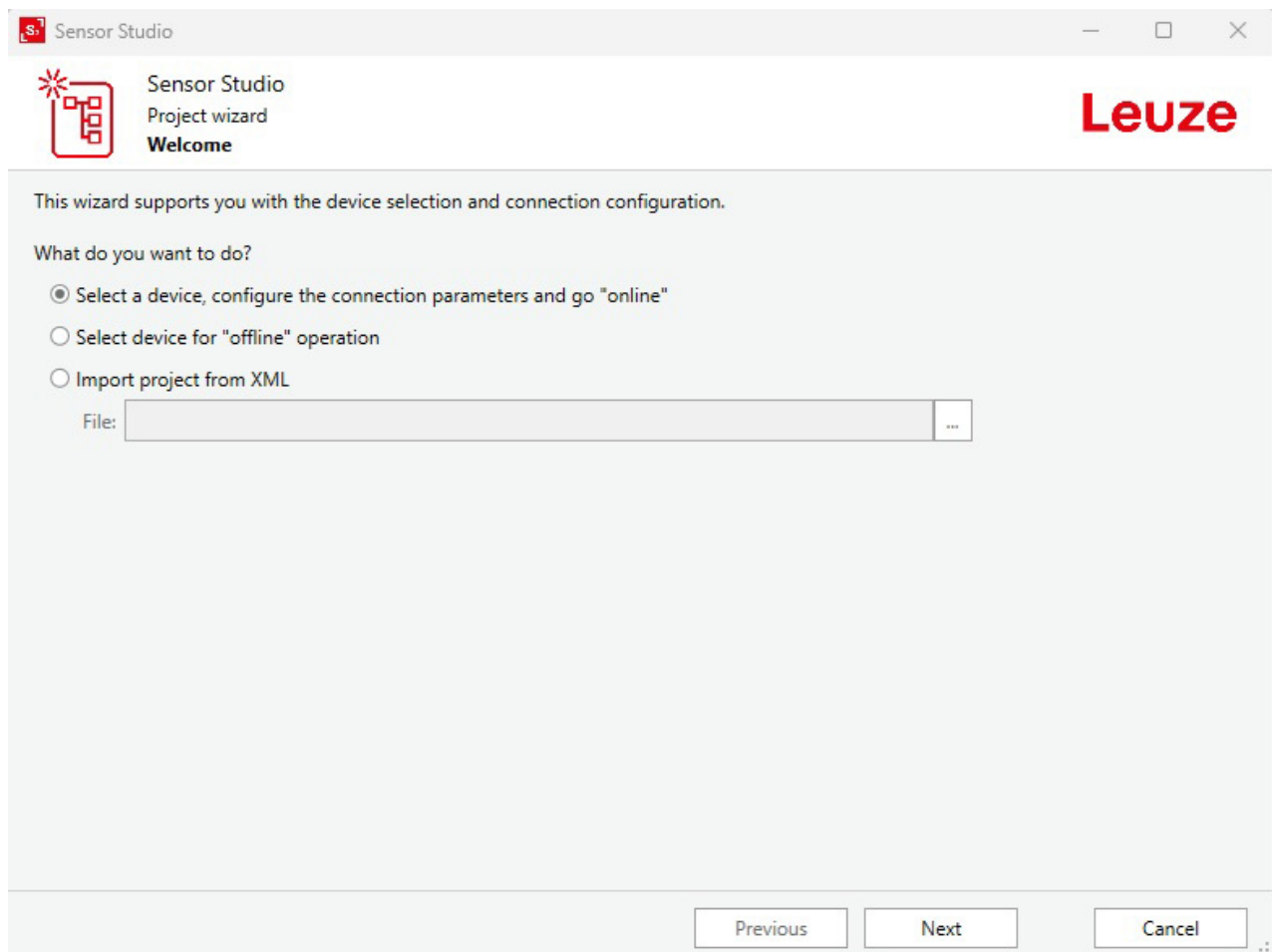
Bild 8.37: Projektassistent starten
