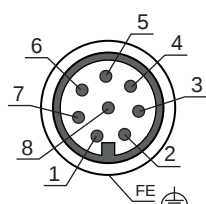
图 7.2: 引脚分配 M12 插头 · 8 针
