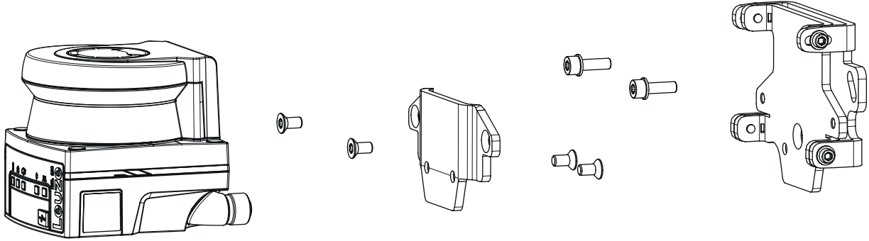
Resim 6.16: Duvar braketini ile montaj
