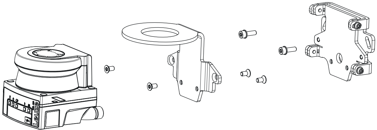
그림 6.17: 벽 홀더 및 보호 브래킷으로 설치
