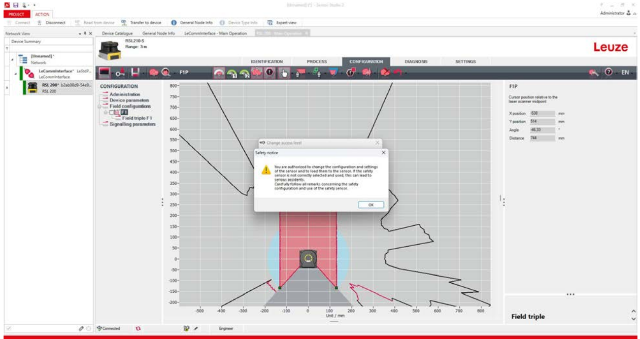
그림 8.39: 안전 구성을 다운로드하기 전 점검
