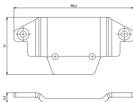
그림 14.4: 설치 시스템 BTU 500M
