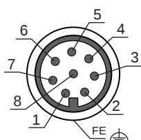
그림 7.2: M12 커넥터(8핀) 핀 지정
