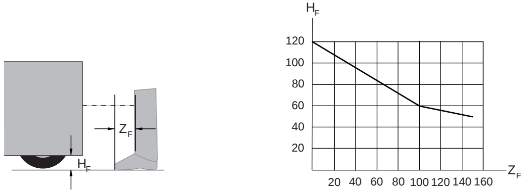
그림 6.14: 바닥의 빈 공간 H_F 가 부족할 때 여유한계 H_F 를 결정하기 위한 도표 차량 높이가 50mm 미만인 경우 항상 추가 거리 Z_F = 150\text{mm} 가 필요합니다. 바퀴가 측벽 근처에 장착되어 있는 경우, 여유한계 Z_F > 150\text{mm} 를 항상 합산하십시오.
