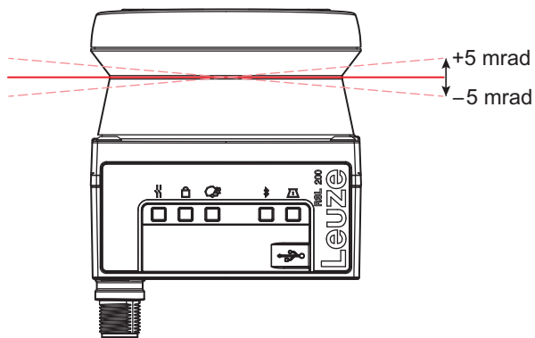
그림 14.2: 기울기 오차
