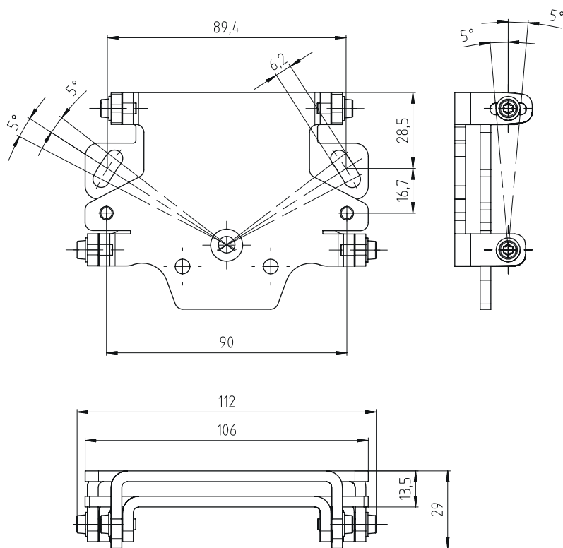
그림 14.4: 설치 시스템 BTU 500M
