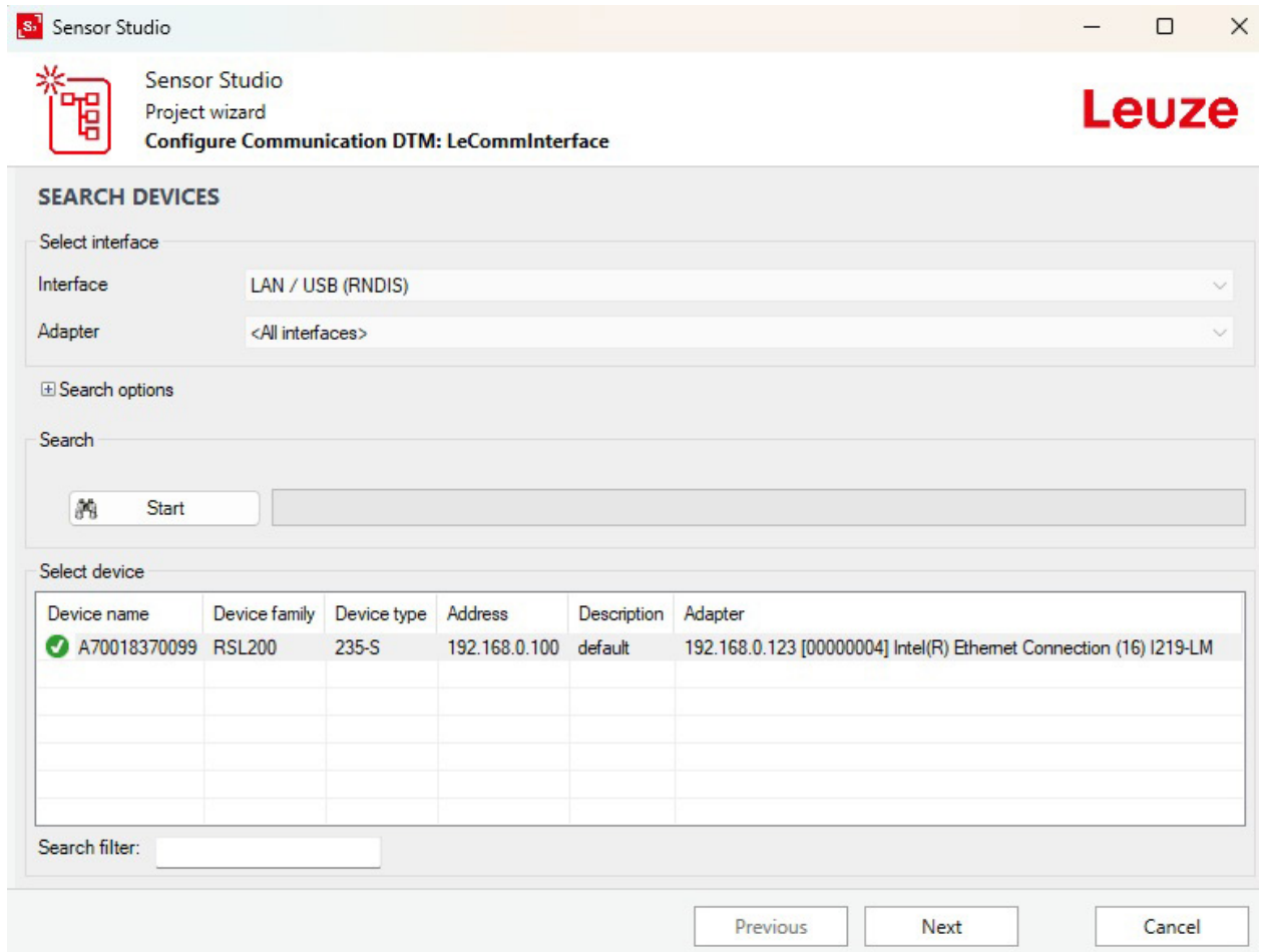
그림 8.3: 프로젝트 도우미에서 장치 선택
