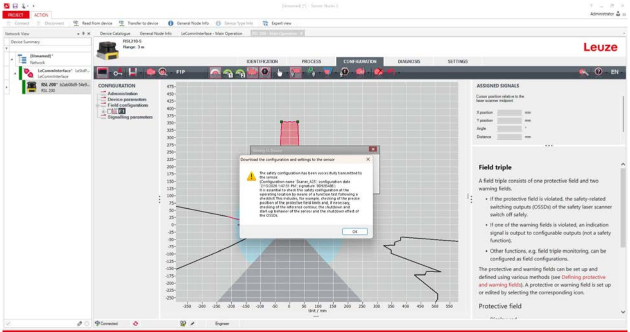
그림 8.40: 확인: 안전 구성이 다운로드됨
