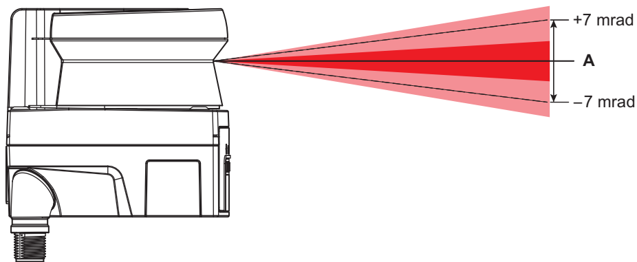
그림 14.3: 원뿔 오차
