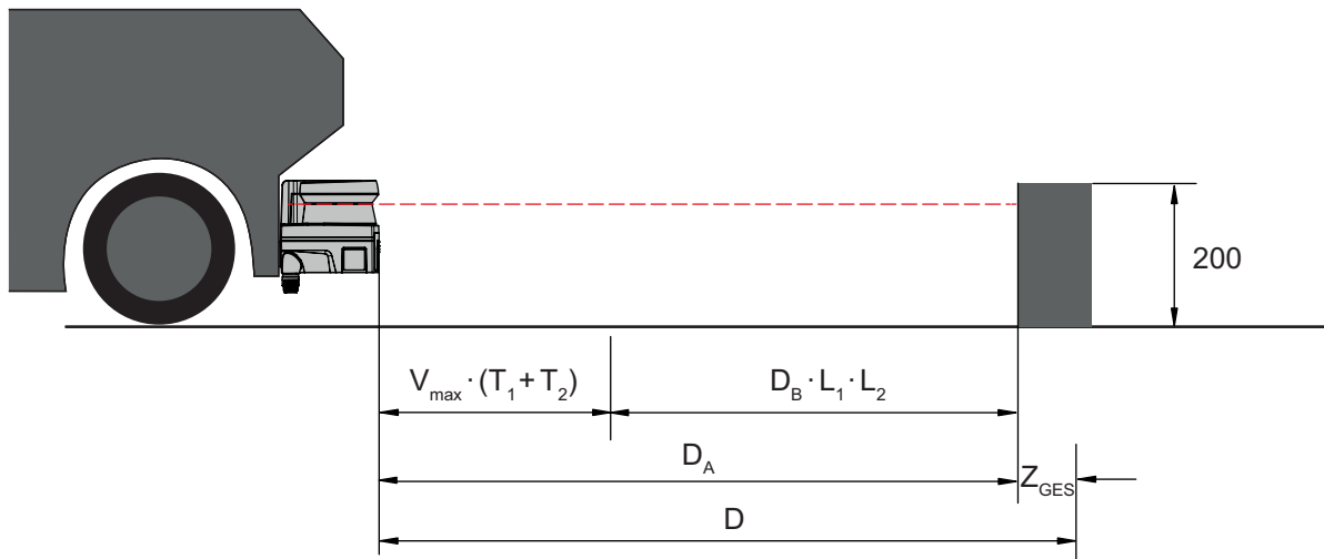
그림 6.13: 모바일 위험구역 안전장치, 필요한 최소 간격 D의 계산
