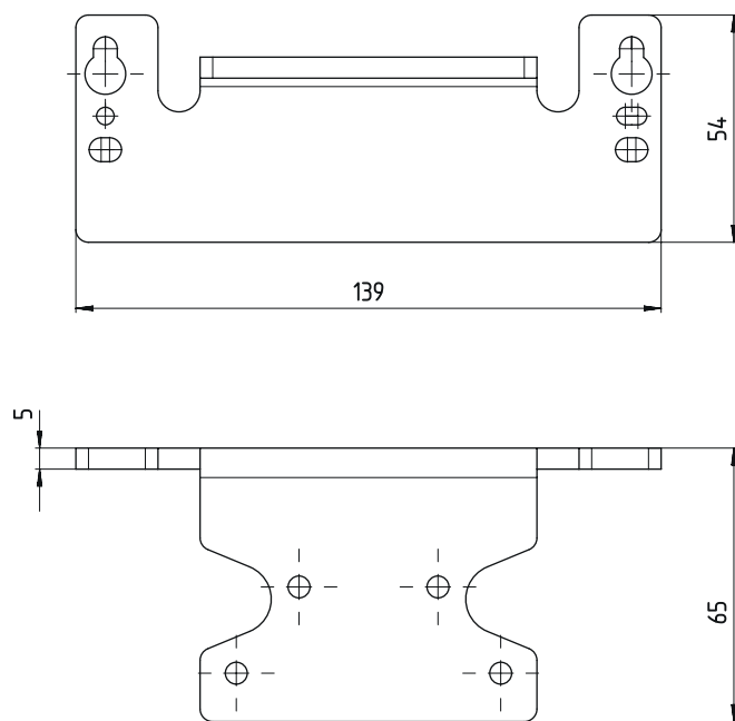
그림 14.6: 보호 브래킷 BTP 500M
