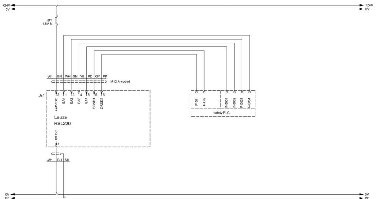
그림 7.3: RSL 220, 안전 제어 장치 포함
