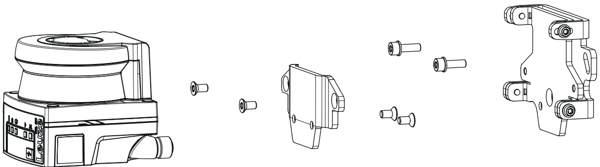
그림 6.16: 벽 홀더로 설치
