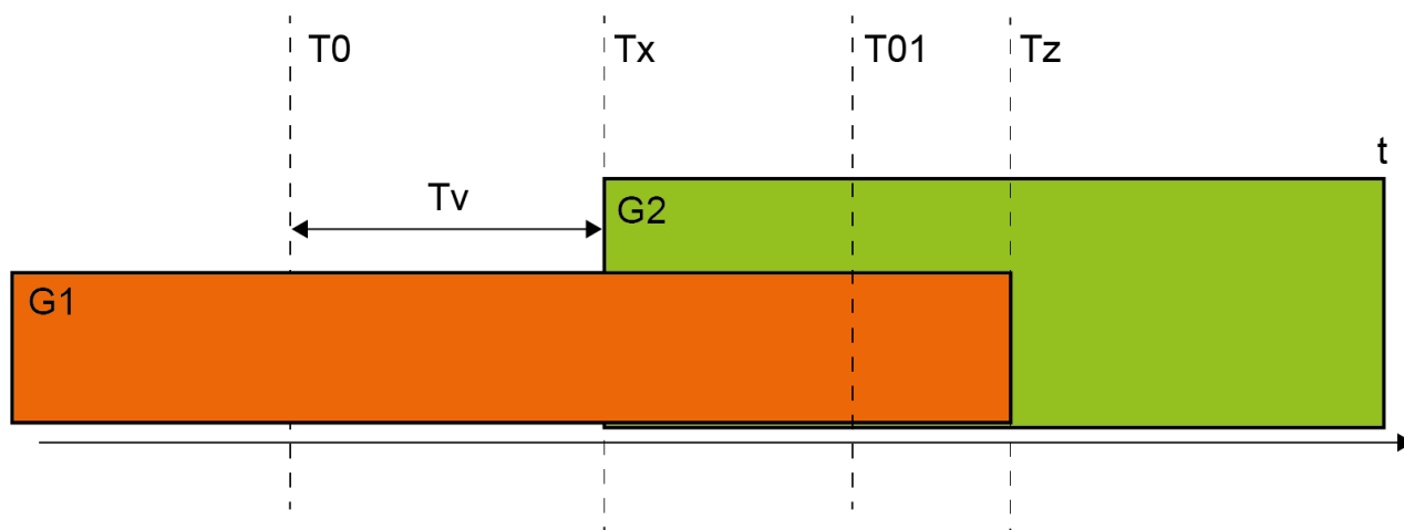
Figura 4.7: Commutazione delle coppie di campi con 2 punti pericolosi
