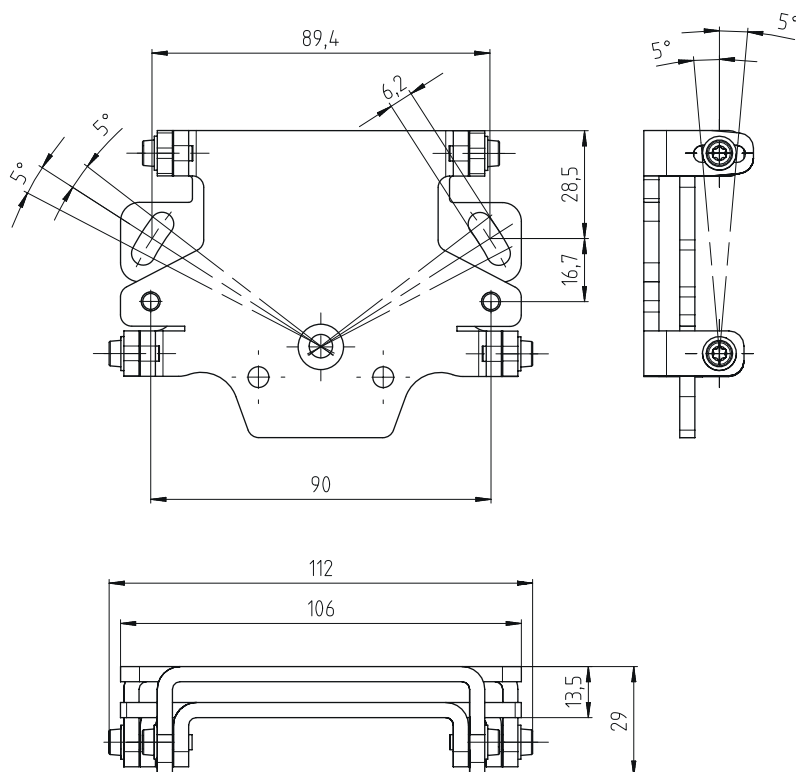
Figura 14.4: Sistema di montaggio BTU 500M
