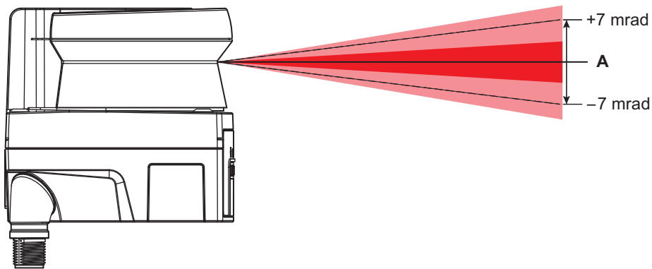
Bild 14.3: Kegelfehler
