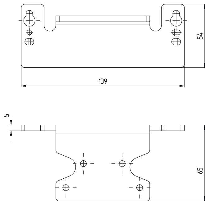
Bild 14.6: Schutzbügel BTP 500M
