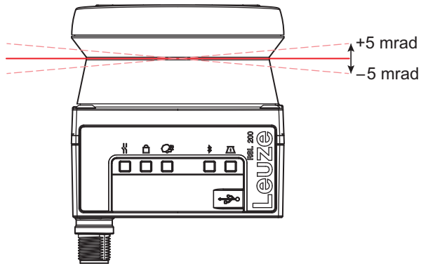
Bild 14.2: Neigungsfehler
