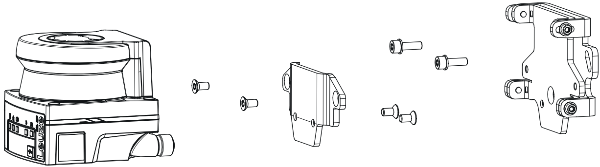
Resim 6.16: Duvar braketi ile montaj
