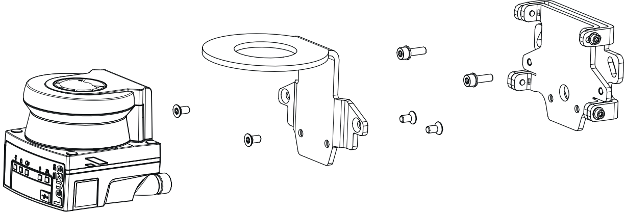
Resim 6.17: Duvar braket ve koruyucu braket ile montaj
