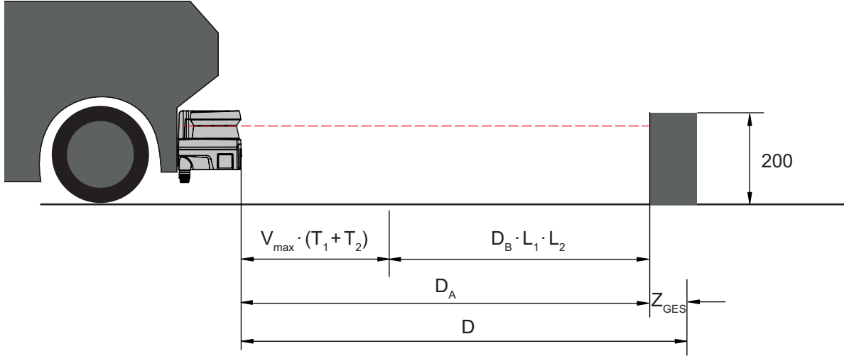
Resim 6.13: Mobil tehlike alanı emniyeti, gerekli asgari mesafe D'nin hesaplanması
