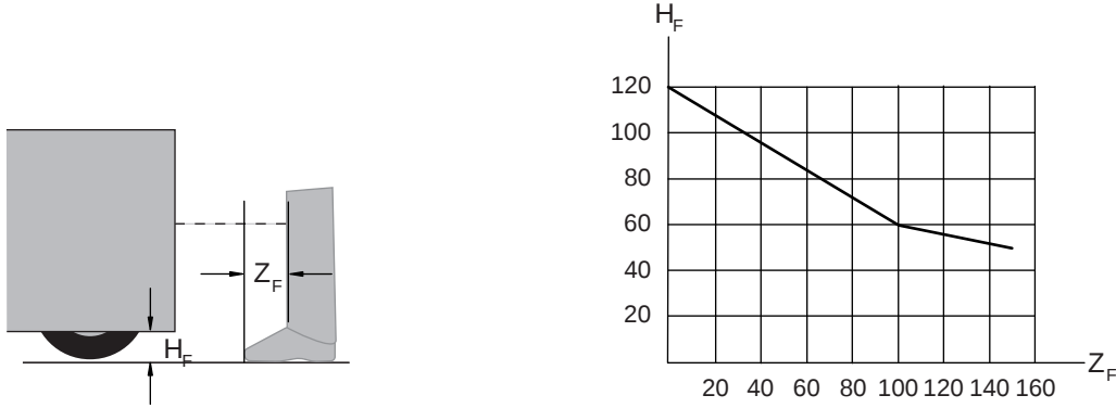
Resim 6.14: İlave yük Z_F 'nin kötü zemin serbestliği H_F 'de belirlenmesi için diyagram
