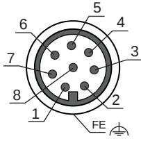
Resim 7.2: M12 konnektörünün pim tahsisi, 8 kutuplu
