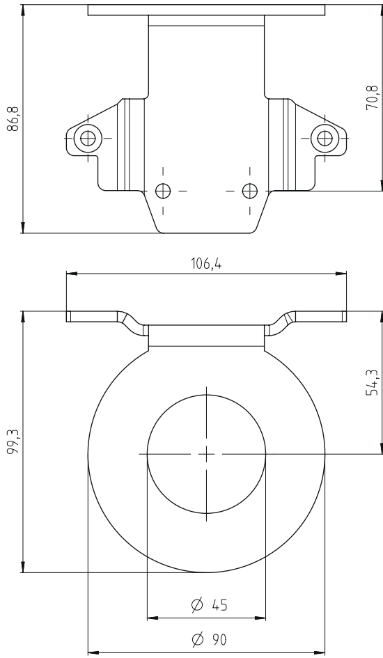
Resim 14.6: Koruma demiri BTP 500M
