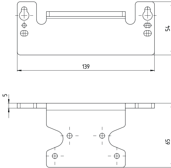
Resim 14.6: Koruma demiri BTP 500M
