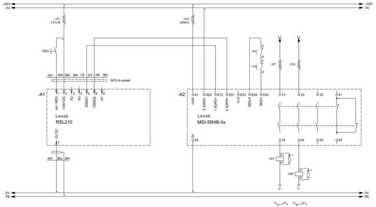
Resim 7.3: RSL 210 ile emniyet rölesi MSI-SR4B-0x
