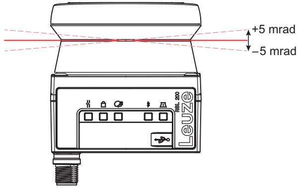
Resim 14.2: Eğim hatası
