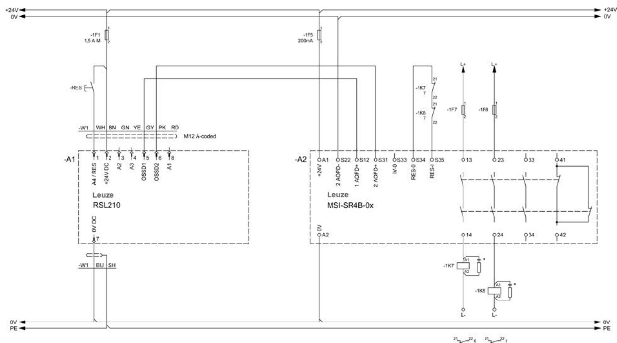
Fig. 7.3: RSL 210 com relé de segurança MSI-SR4B-0x
