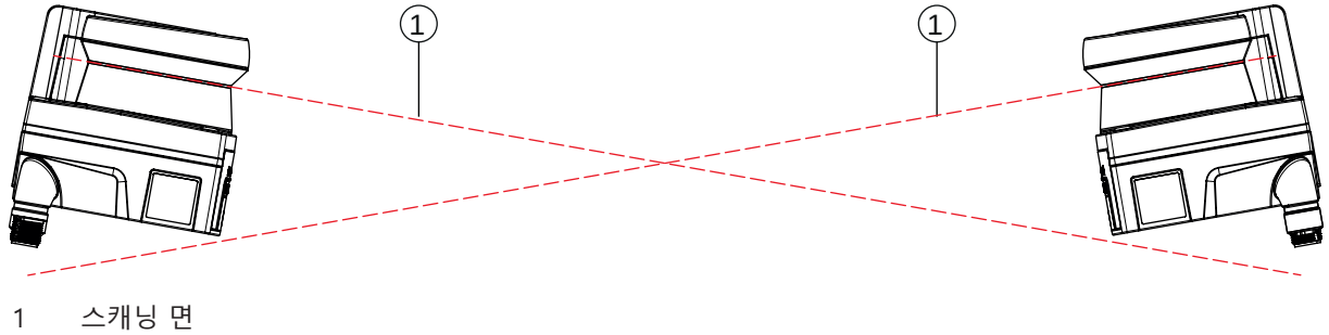
그림 6.9: 마주보고 설치, 높이 차이를 두지 않음. 교차 정렬
