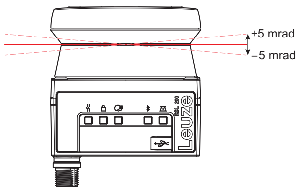
Fig. 14.2: Erreur d'inclinaison
