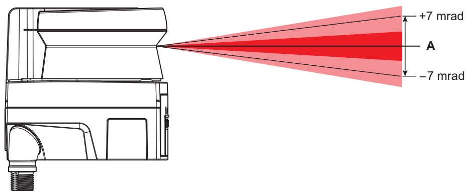
Fig. 14.3: Erreur de cône
