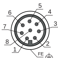
Fig. 7.2: Affectation des broches du connecteur M12 à 8 broches
