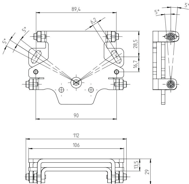
Fig. 14.4: Système de montage BTU 500M
