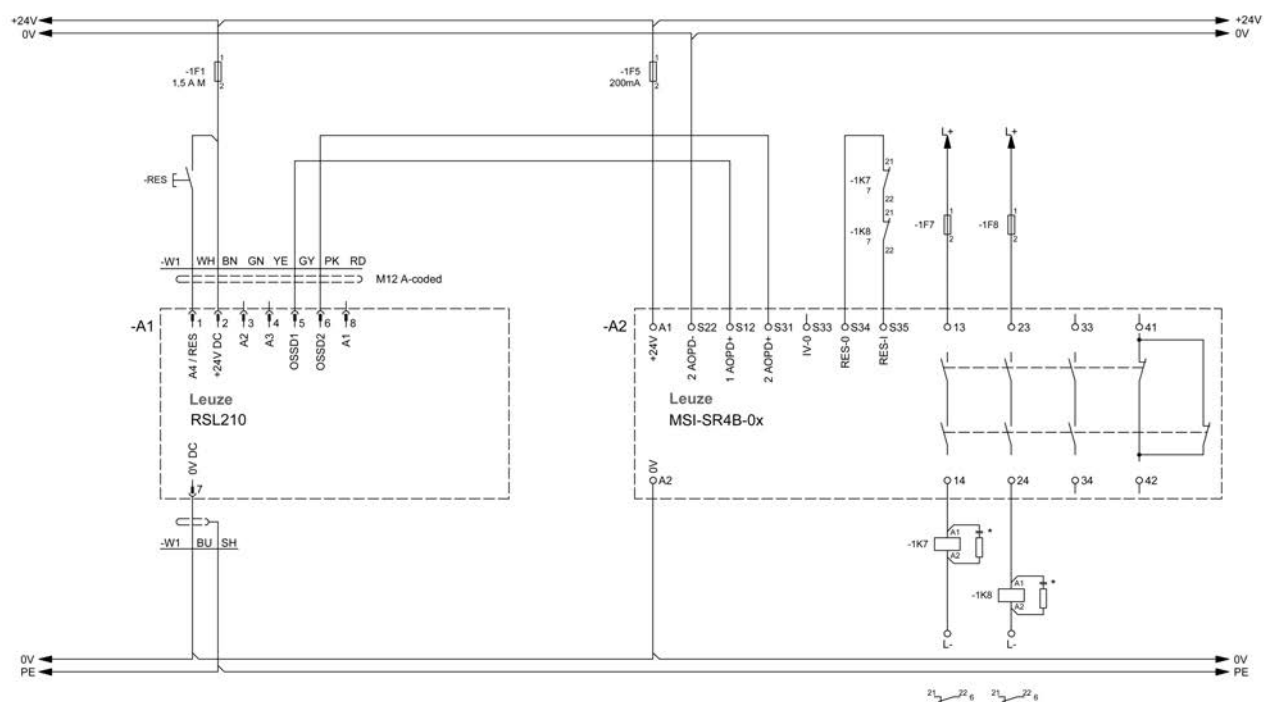
Fig. 7.3: RSL 210 avec relais de sécurité MSI-SR4B-0x
