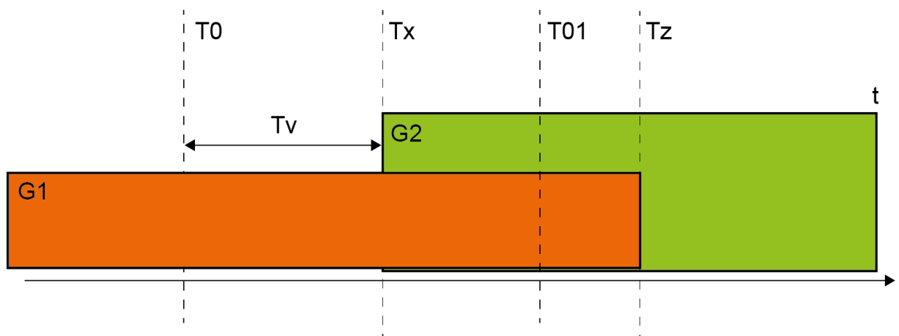
Bild 4.7: Feldpaarumschaltung bei 2 Gefahrenstellen
