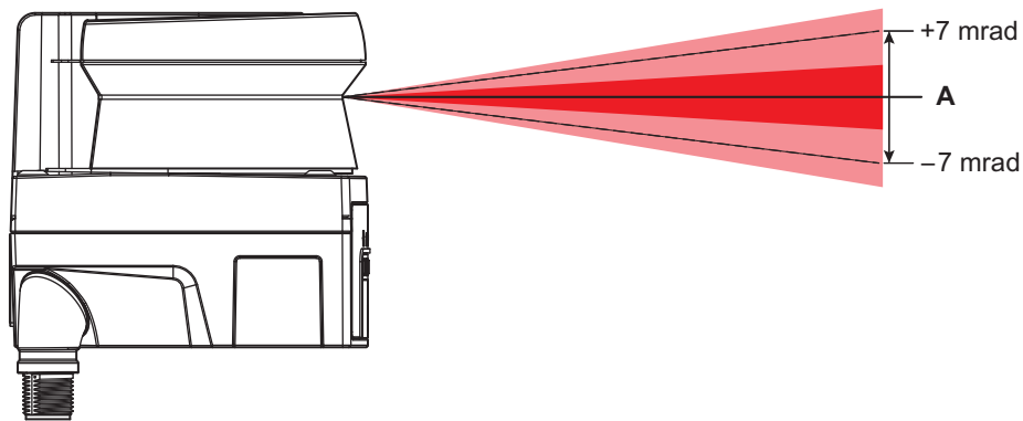
Bild 14.3: Kegelfehler
