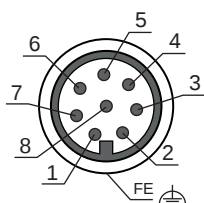
Bild 7.2: Pinbelegung M12-Stecker, 8-polig
