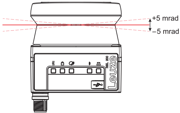
Bild 14.2: Neigungsfehler
