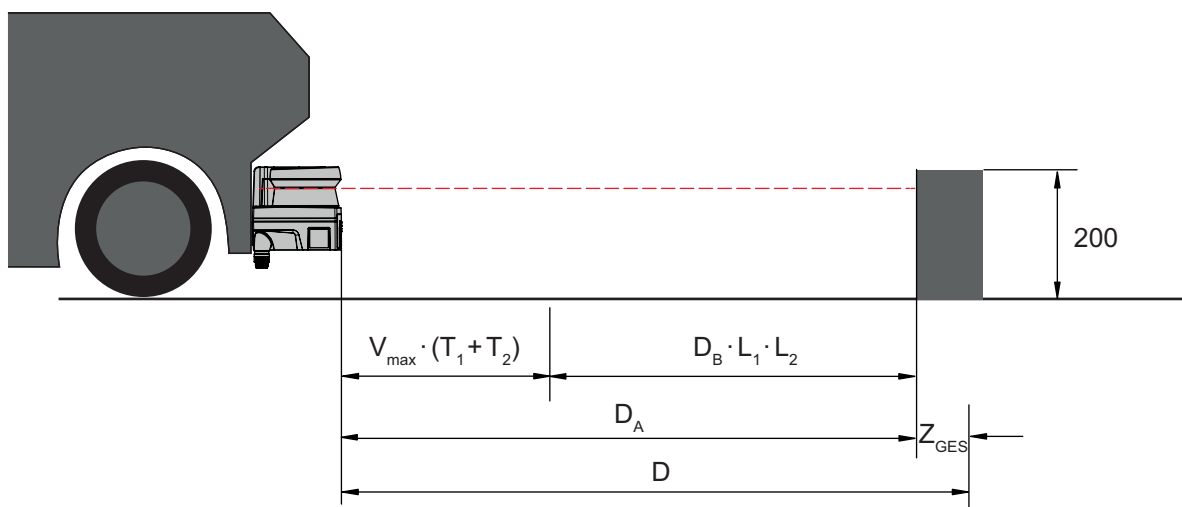
Bild 6.13: Mobile Gefahrbereichssicherung, Berechnung der erforderlichen Mindestdistanz D
