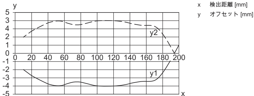
反射率90%の場合の典型的な応答時間 ( 設定距離200 mm )
