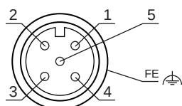
Figura 7.1: Asignación de pines del emisor
