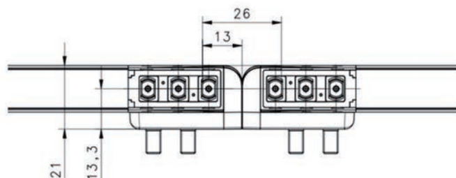
Figura 6.14: Fijación con soportes de montaje L
