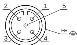
Figura 7.2: Asignación de pines del receptor
