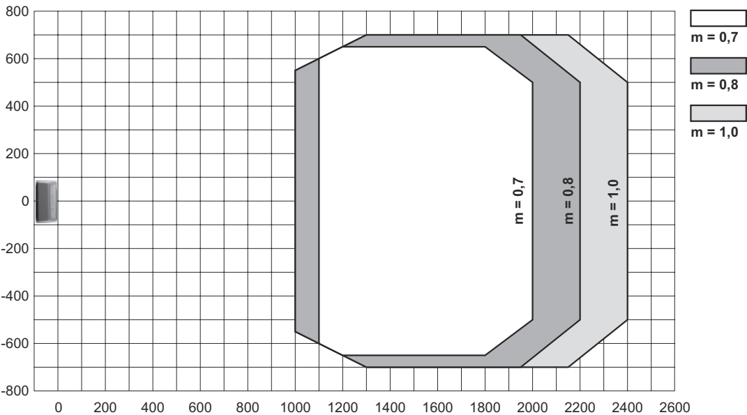
Curva del campo de lectura
