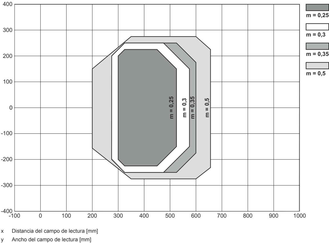
Curva del campo de lectura
