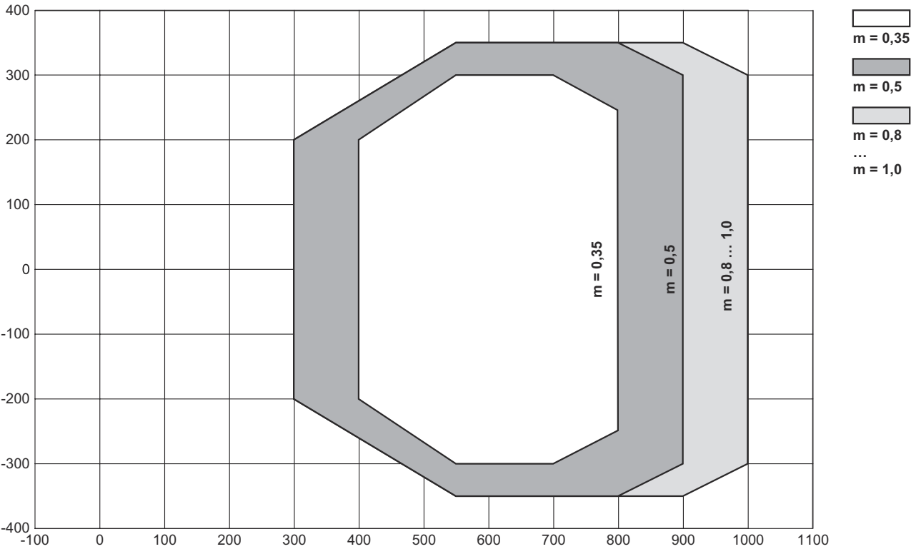
Curva del campo de lectura
