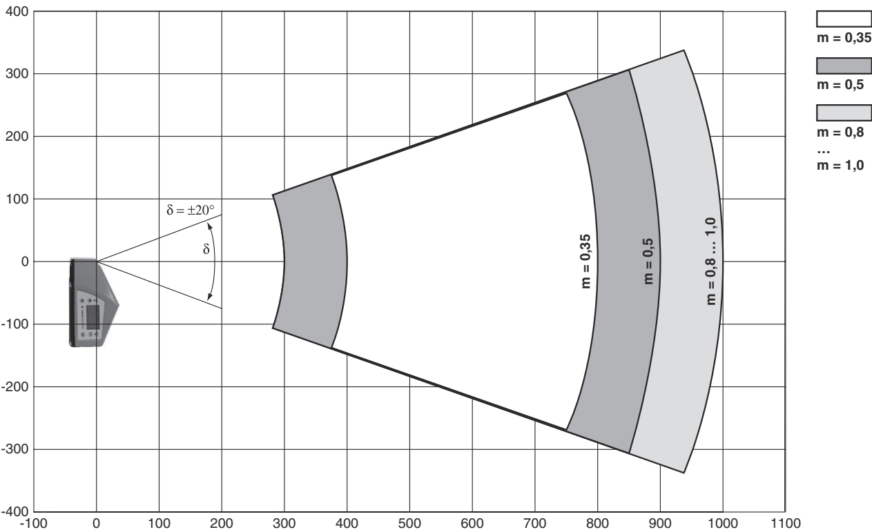
Curva lateral del campo de lectura
