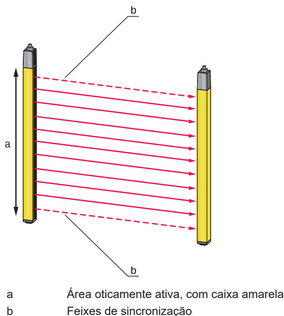
Fig. 3.1: Sistema transmissor/receptor
