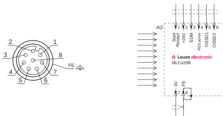
Fig. 7.3: Affectation des broches et schéma de raccordement du récepteur
