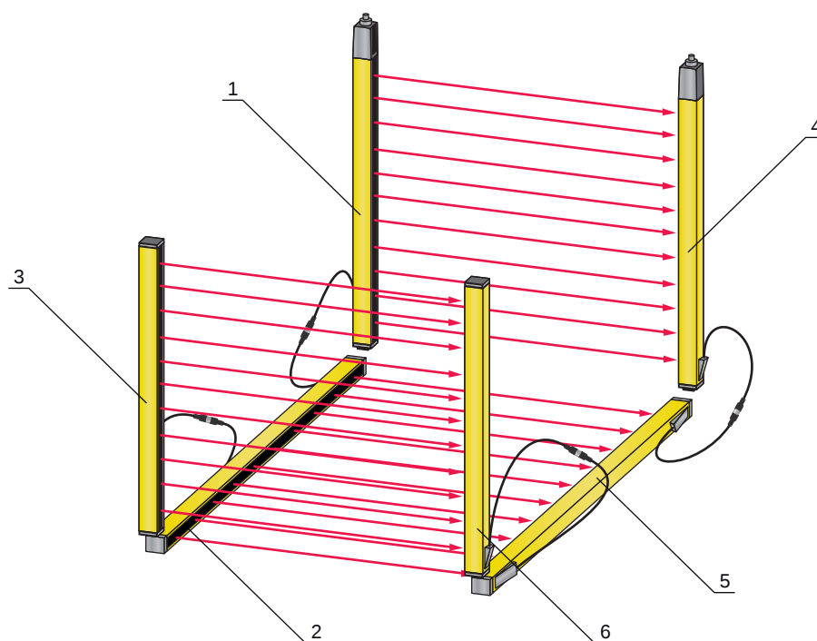
Fig. 3.3: Système en cascade avec 2 barrières immatérielles de sécurité MLC
