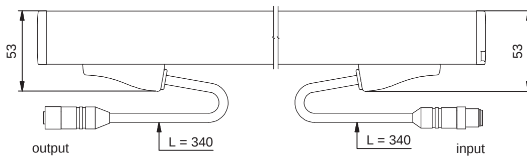
Fig. 14.1: Dimensions de l'émetteur Host et du récepteur Host
