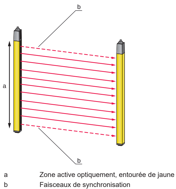
Fig. 3.1: Système émetteur-récepteur
