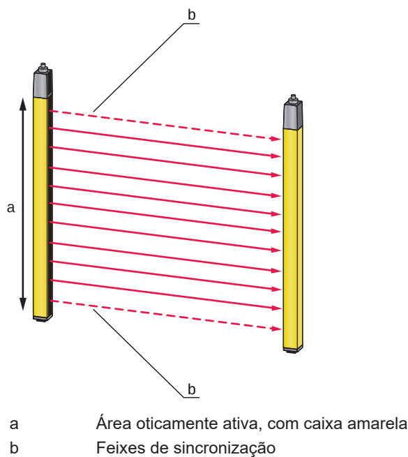
Fig. 3.1: Sistema transmissor/receptor
