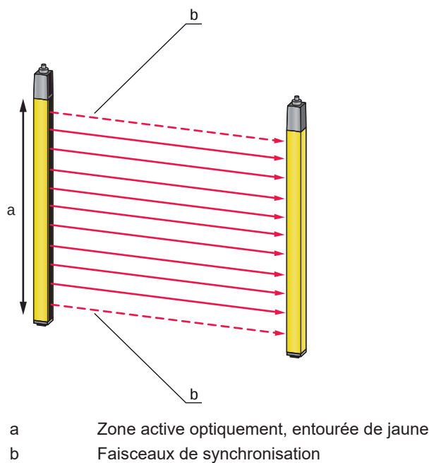
Fig. 3.1: Système émetteur-récepteur
