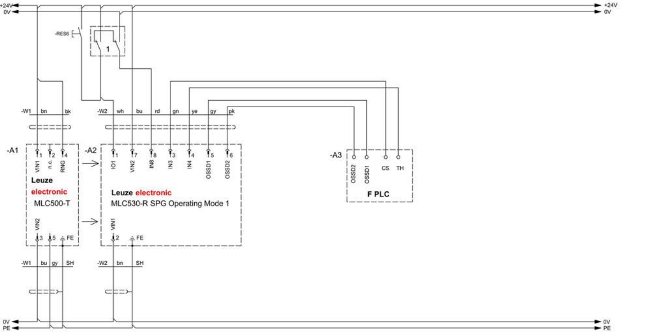
Figura 8.4: Modo de trabajo 1: ejemplo de conexión con Smart Process Gating (SPG)
