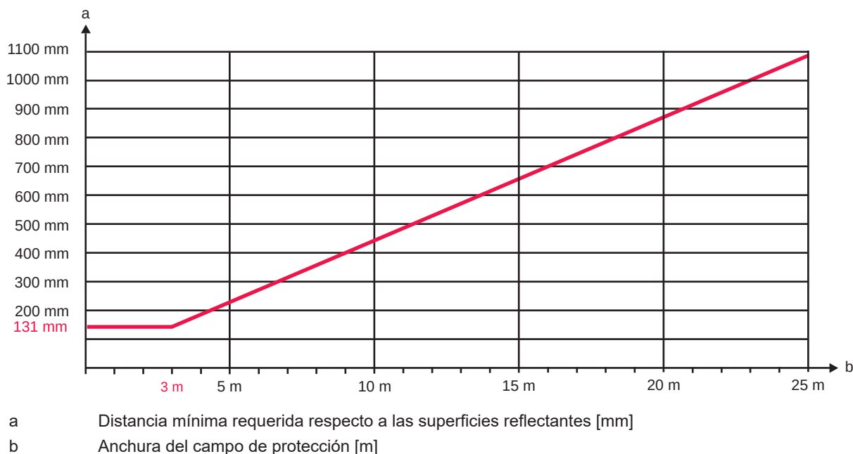
Figura 7.3: Distancia mínima respecto a las superficies reflectantes en función de la anchura del campo de protección
