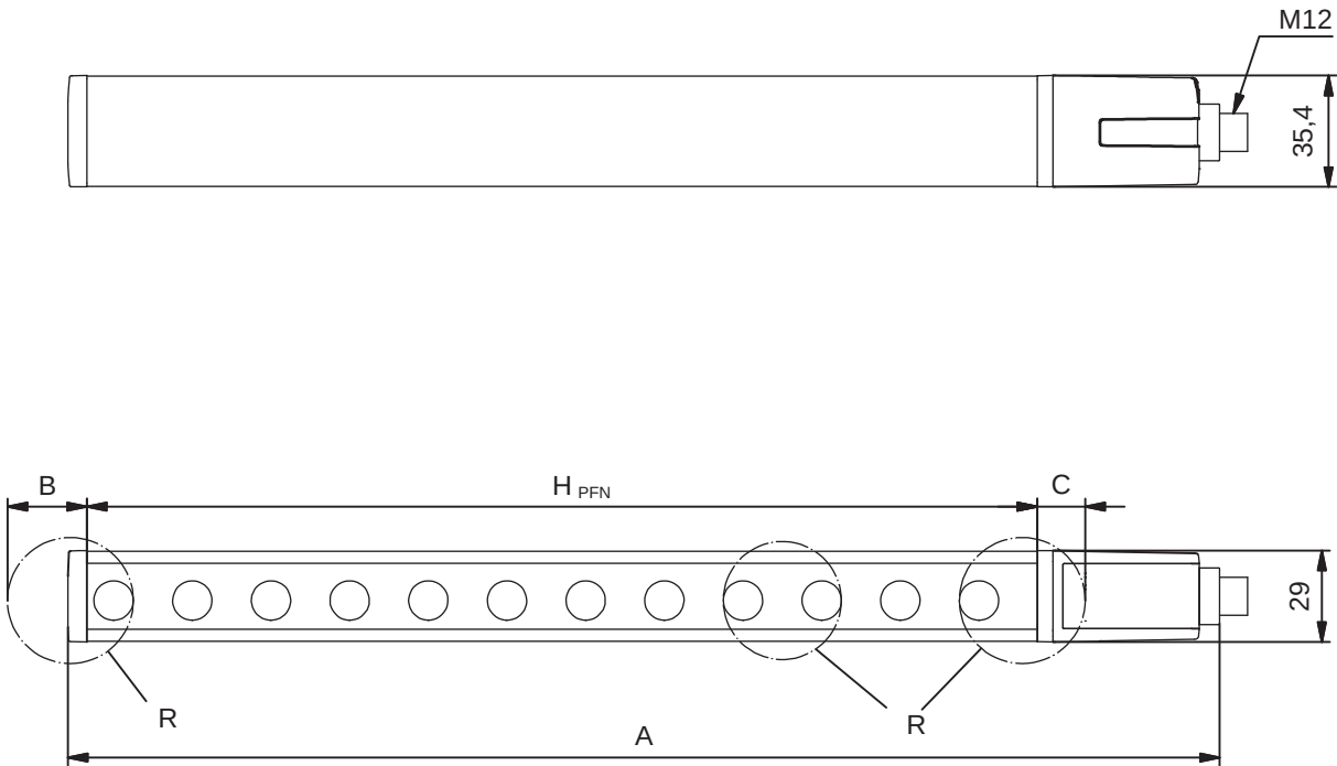
Figura 15.1: Medidas del emisor y receptor La altura del campo de protección efectiva H_{PFE} sale de las medidas del área óptica hasta los bordes exteriores de los círculos marcados con R.
