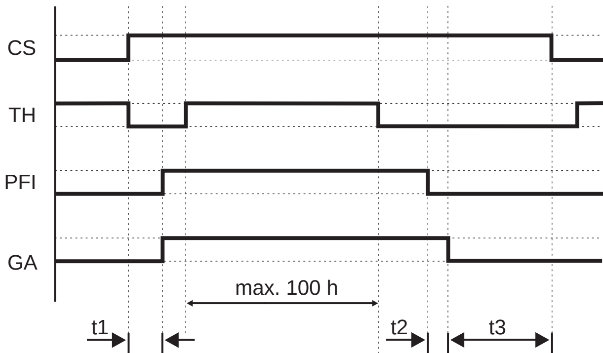
Figura 4.10: Prolongación del timeout de SPG
