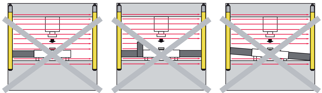
Figura 5.3: Blanking fijo: prevención de «formación de sombras»
