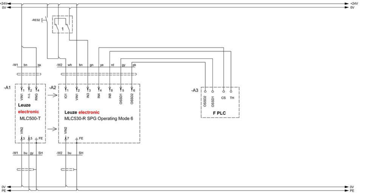
Figura 8.7: Modo de trabajo 6: ejemplo de circuito con Smart Process Gating (SPG)
