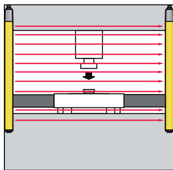
Figura 5.2: Blanking fijo: los bloqueos mecánicos evitan la intervención lateral en el campo de protección
