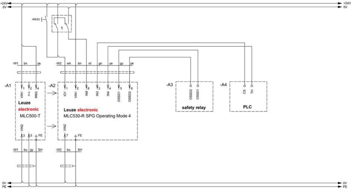
Figura 8.5: Modo de trabajo 4: ejemplo de circuito con Smart Process Gating (SPG)
