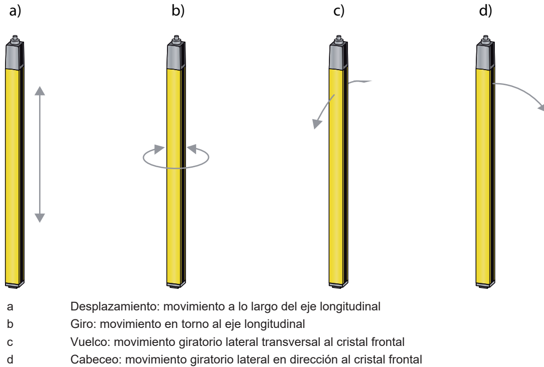
Figura 7.6: Direcciones del movimiento en la alineación del sensor de seguridad
