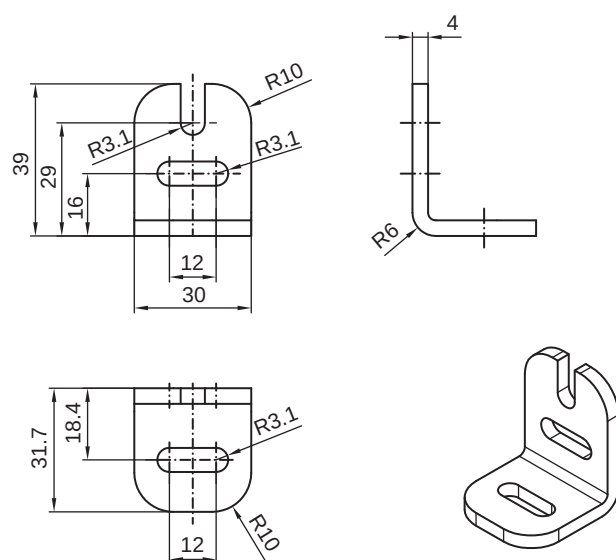
Figura 15.3: Soporte angular BT-L
