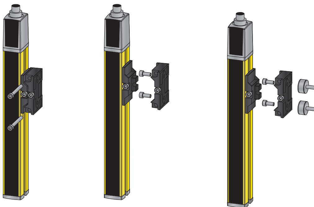
Figura 7.9: Montaje a través de soporte orientable BT-2SB10
