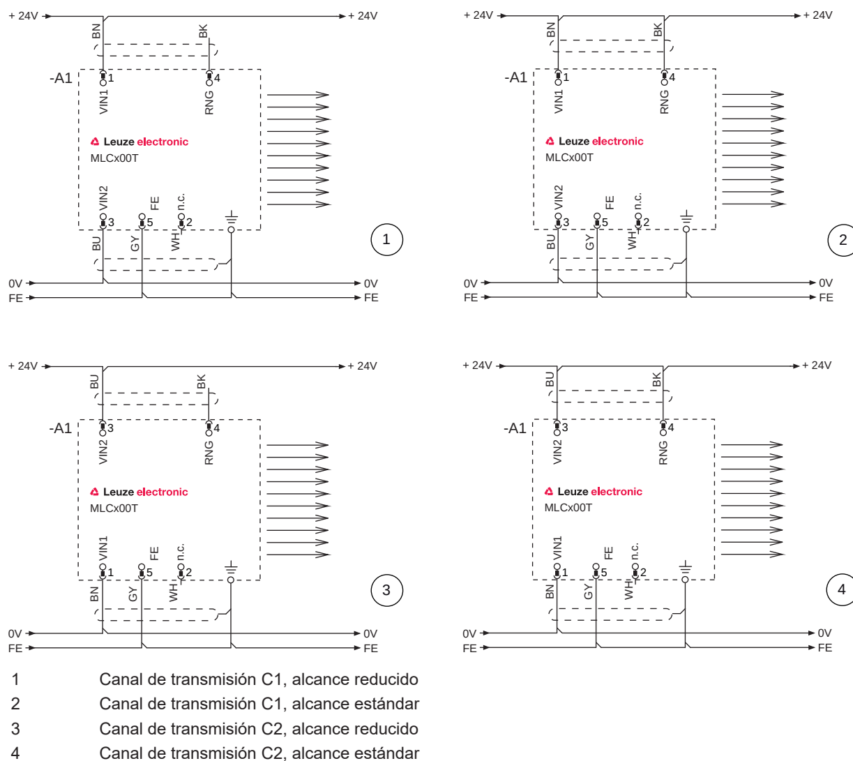
Figura 8.2: Ejemplos de conexión del emisor
