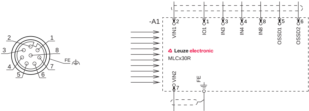
Figura 8.3: Asignación de pines y esquema de conexiones del receptor
