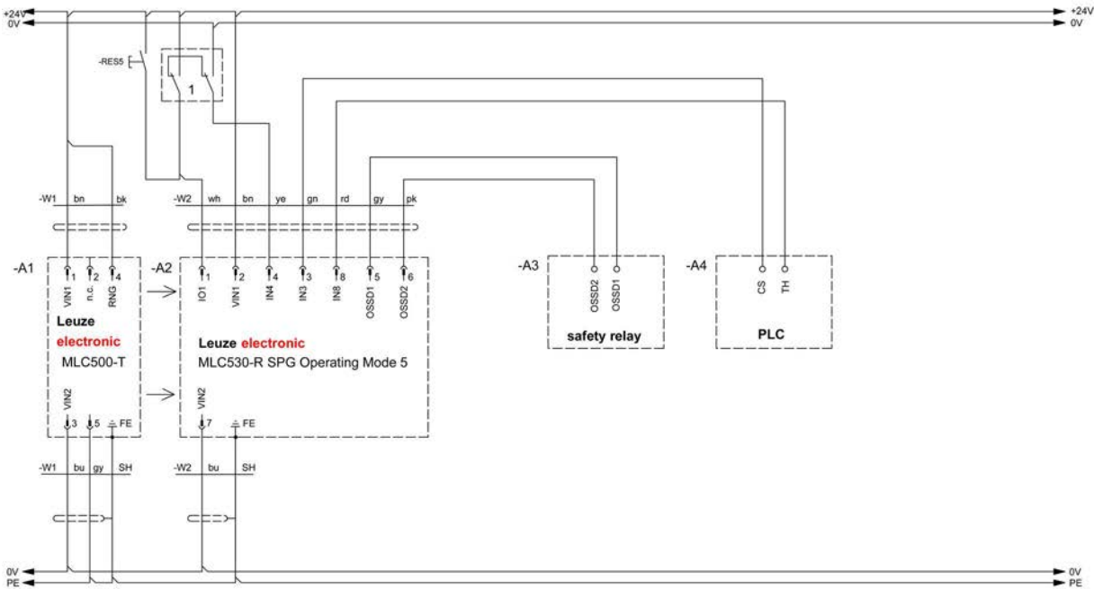
Figura 8.6: Modo de trabajo 5: ejemplo de circuito con Smart Process Gating (SPG)
