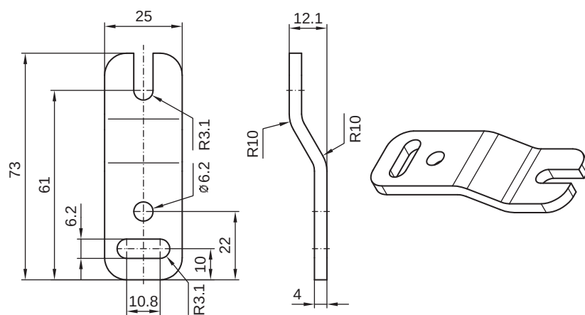
Figura 15.4: Soporte paralelo BT-Z
