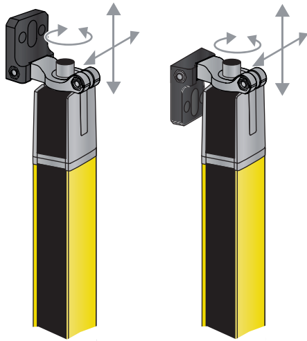
Figura 7.8: Montaje mediante soporte giratorio BT-2HF
