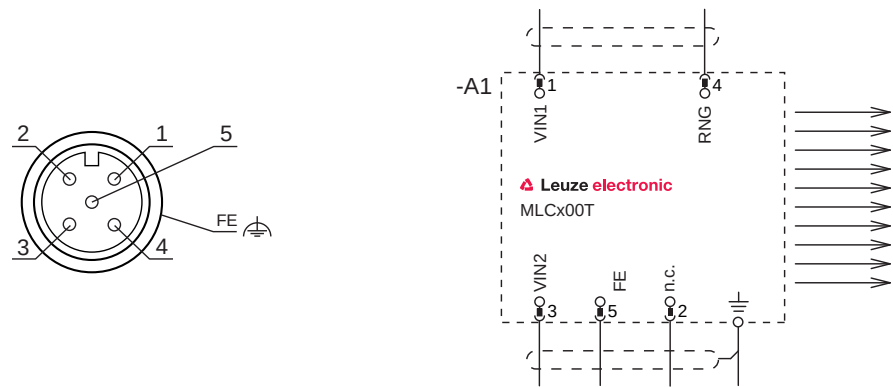
Figura 8.1: Asignación de pines y esquema de conexiones del emisor
