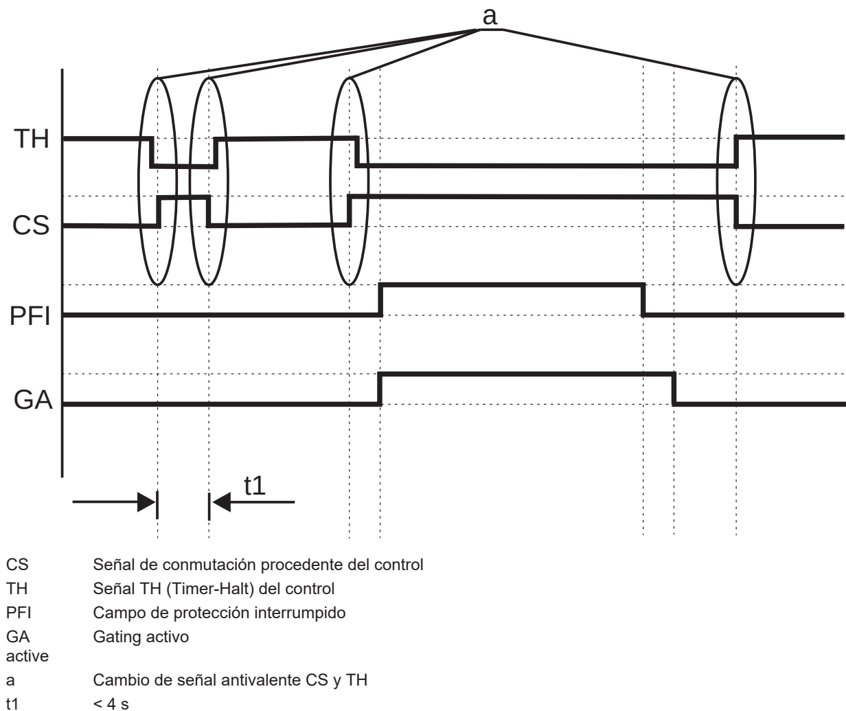
Figura 4.4: Modo de trabajo 1 - Stop cualificado
