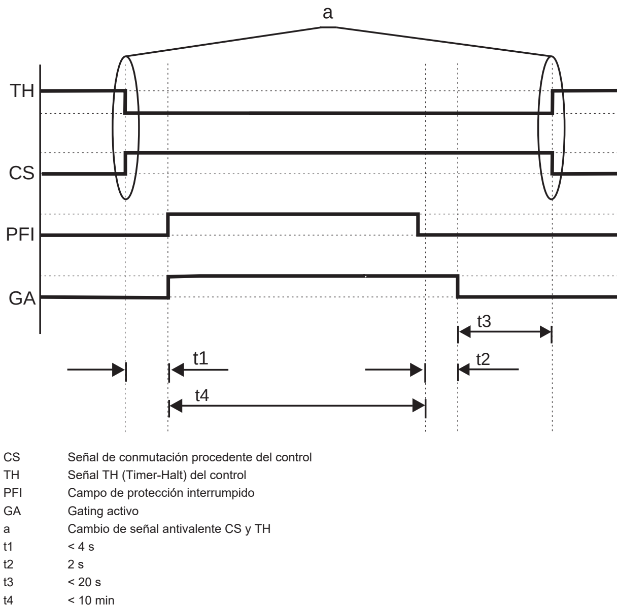
Figura 4.3: Modo de trabajo 1 - Stop cualificado
