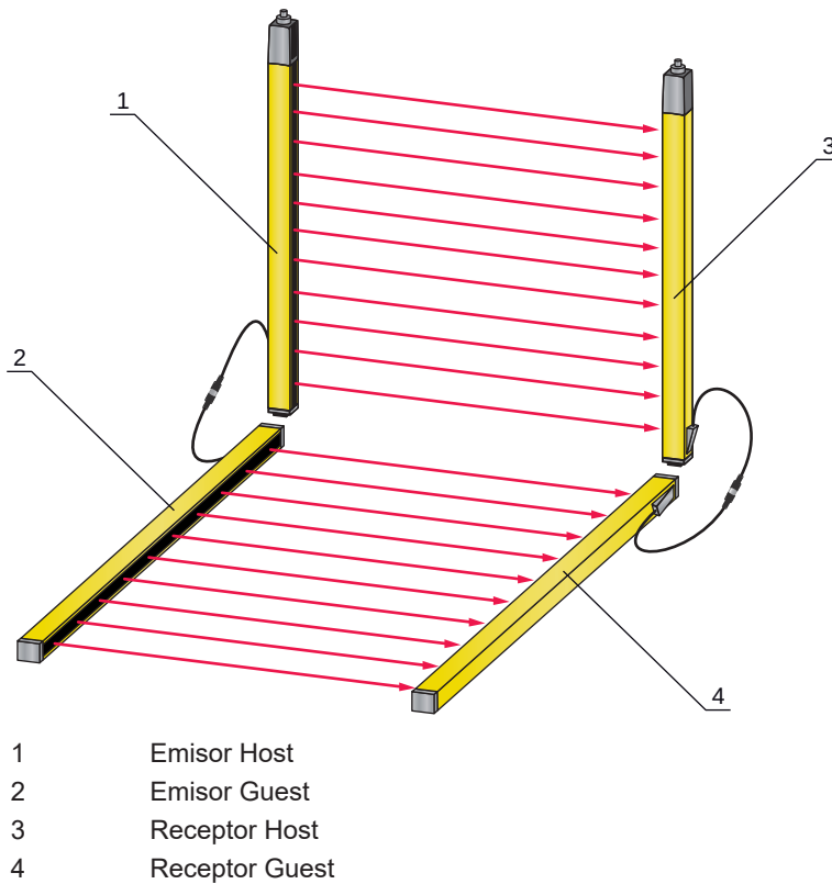
Figura 3.3: Sistema en cascada con 2 cortinas ópticas de seguridad MLC
