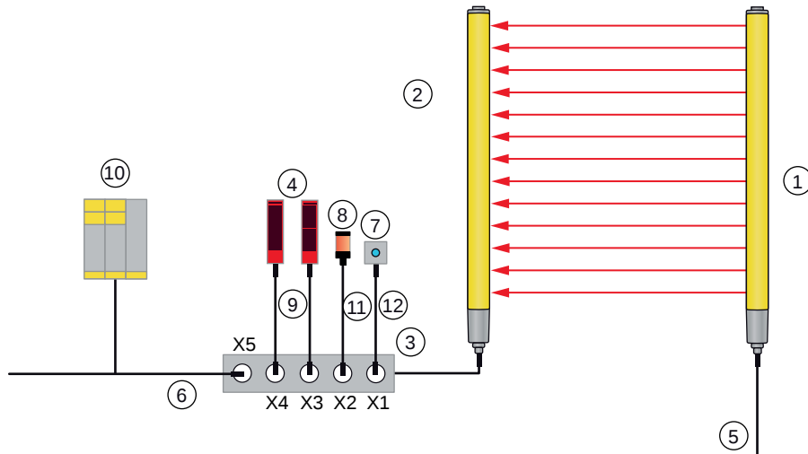
Figura 7.14: Modo de funcionamiento 6: ejemplo de conexión con muting de 2 sensores con control temporizado (parcial), con unidad de uso y lámpara de muting
