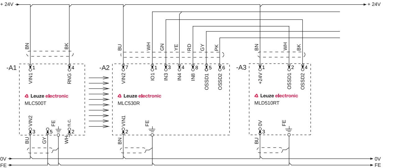
Figura 7.7: Modo de trabajo 2: ejemplo de circuito para encadenar salidas de seguridad electrónicas para la supervisión combinada de accesos y zonas
