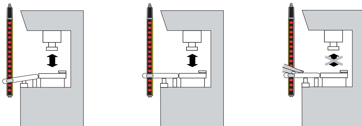
Figura 4.3: Blanking flotante
