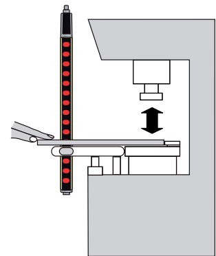
Figura 4.4: Reducción de resolución; varios objetos suficientemente pequeños pueden moverse al mismo tiempo en el campo de protección o eliminarse
