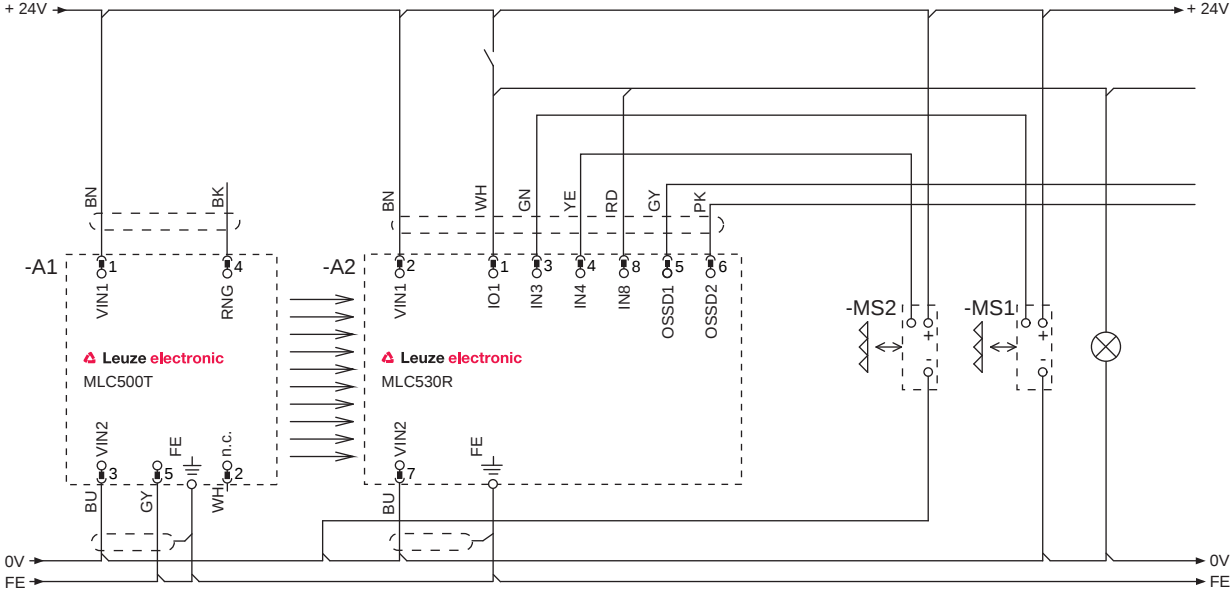
Figura 7.11: Modo de funcionamiento 4: ejemplo de circuito para muting de 2 sensores con control temporizado
