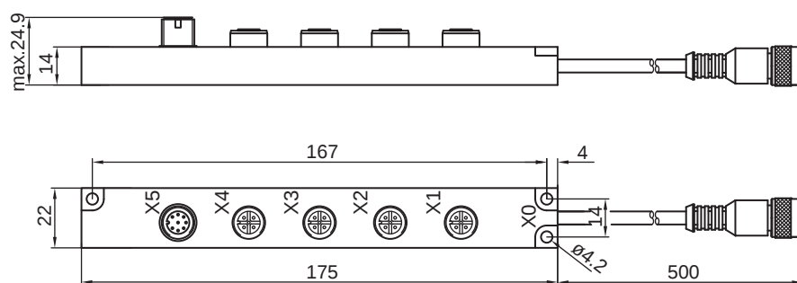
Figura 14.7: Unidad de conexión del sensor AC-SCM8
