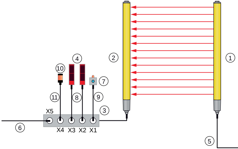
Figura 7.12: Modo de funcionamiento 4: ejemplo de conexión para muting de 2 sensores con control temporizado con unidad de uso
