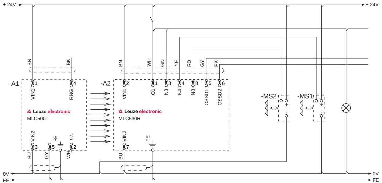
Figura 7.13: Modo de funcionamiento 6: ejemplo de circuito para muting de 2 sensores con control temporizado (parcial)
