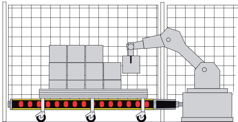
Figura 4.4: Reducción de resolución; varios objetos suficientemente pequeños pueden moverse al mismo tiempo en el campo de protección o eliminarse
