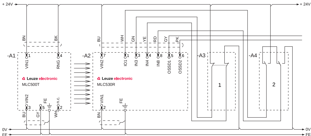
Figura 7.4: Modo de trabajo 1: ejemplo de circuito para encadenar con un interruptor de posición para supervisar la presencia de piezas de máquina con blanking fijo
