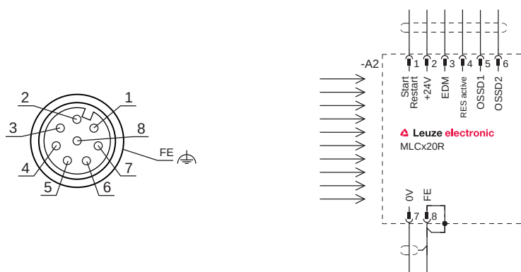
Bild 7.3: Pinbelegung und Anschlussbild Empfänger
