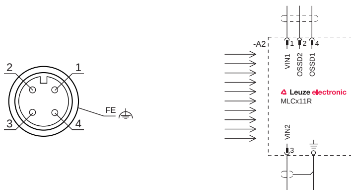
Bild 7.3: Pinbelegung und Anschlussbild Empfänger
