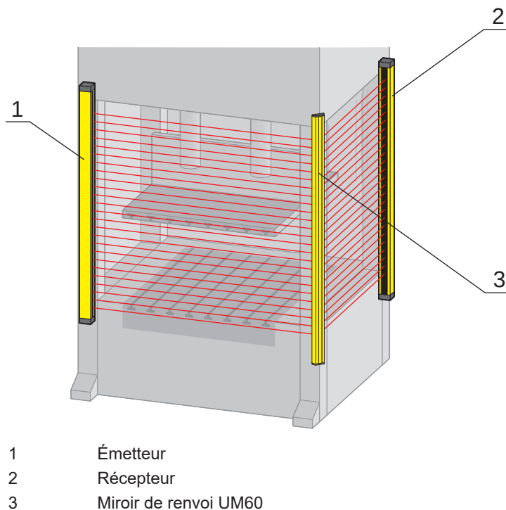
Fig. 6.11: Disposition avec miroir de renvoi pour la sécurisation bilatérale d'un poste dangereux
