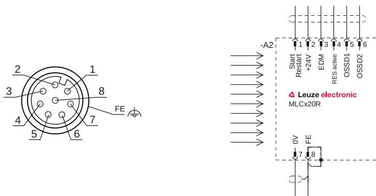
Figura 7.3: Asignación de pines y esquema de conexiones del receptor
