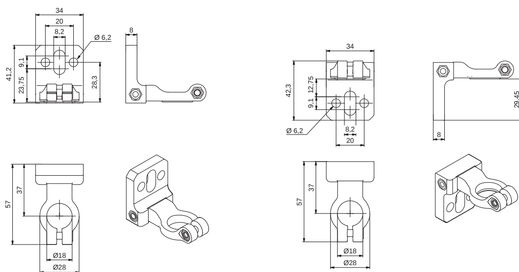
Bild 14.6: Drehhalterung BT-2HF
