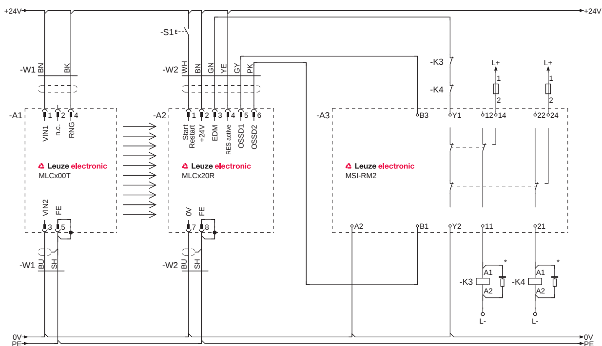
Bild 7.5: Schaltungsbeispiel mit nachgeschaltetem Sicherheits-Schaltgerät MSI-RM2
