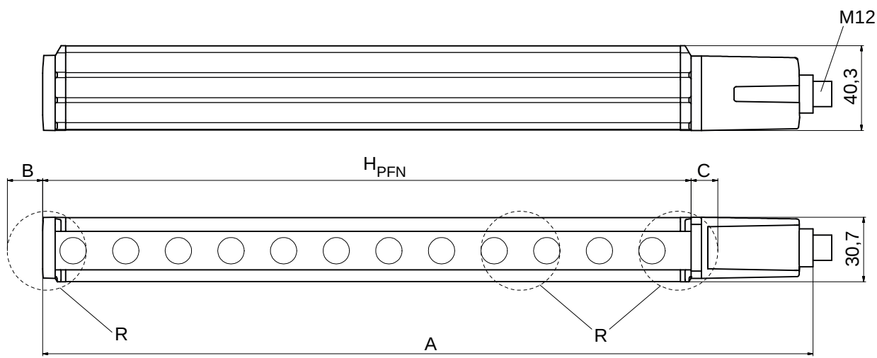
Bild 14.1: Maße Sender und Empfänger Die effektiv wirksame Schutzfeldhöhe H_{PFE} geht über die Maße des Optikbereichs hinaus bis zu den äußeren Rändern der mit R gekennzeichneten Kreise.
