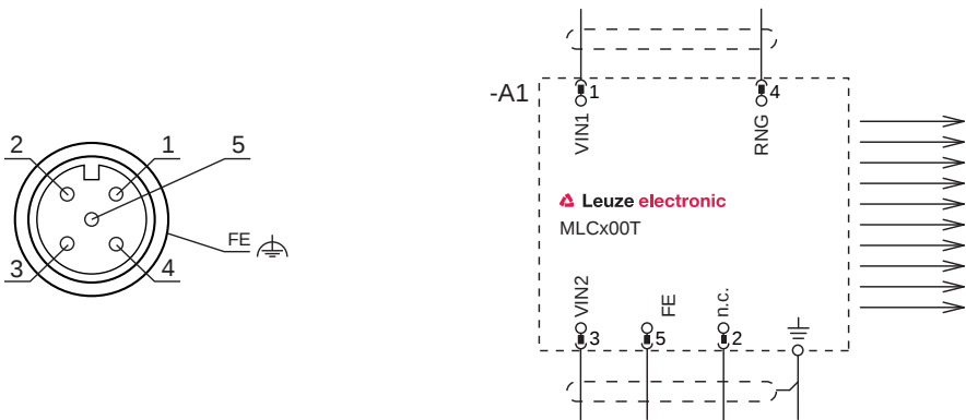
Bild 7.2: Pinbelegung und Anschlussbild Sender
