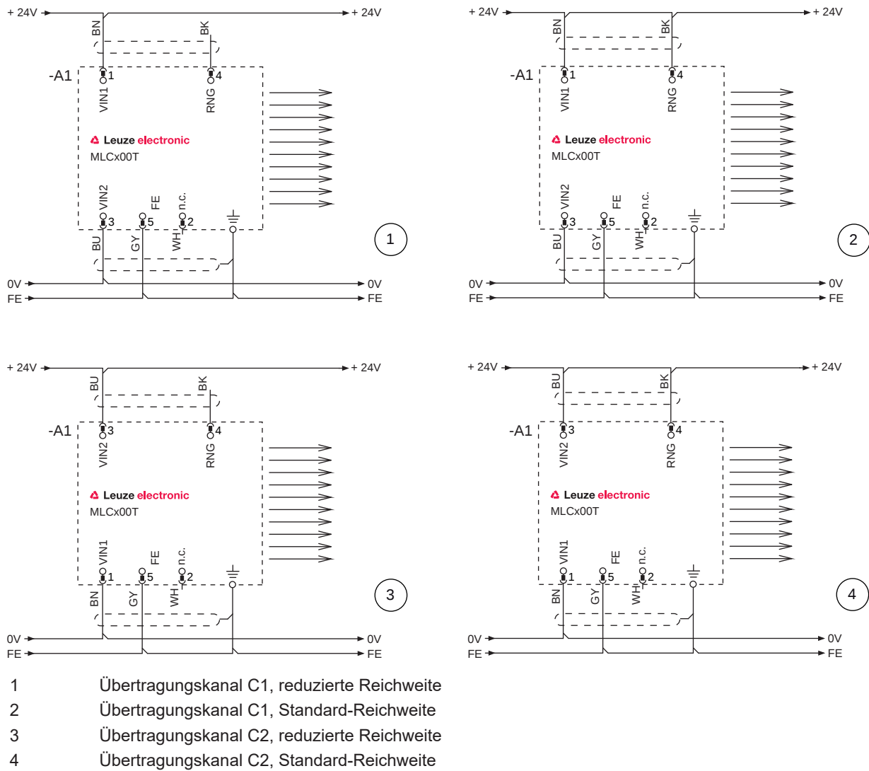
Bild 7.3: Anschlussbeispiele Sender
