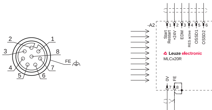
Bild 7.4: Pinbelegung und Anschlussbild Empfänger
