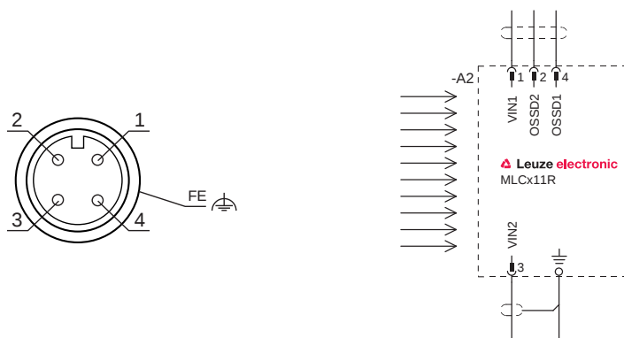
Fig. 7.3: Affectation des broches et schéma de raccordement du récepteur
