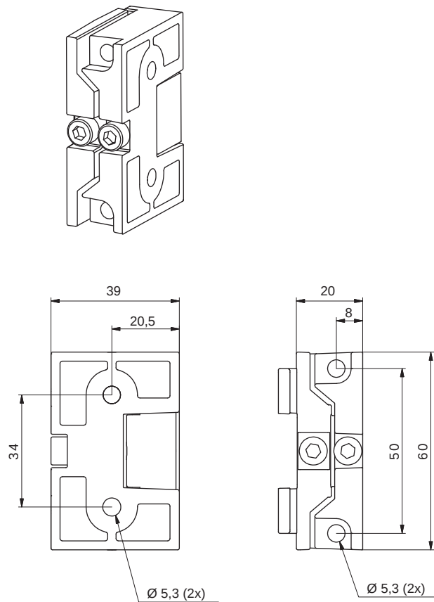
Bild 14.6: Schwenkhalterung BT-2SB10
