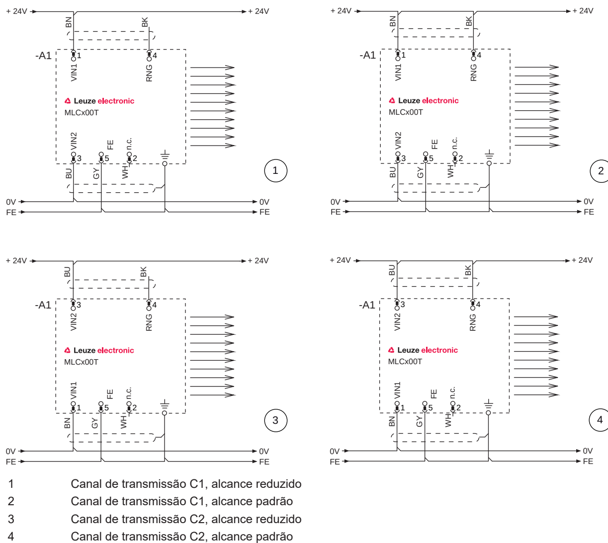
Fig. 7.3: Exemplos de conexão do transmissor
