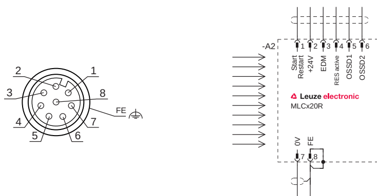
Fig. 7.4: Ocupação de pinos e diagrama de conexões do receptor
